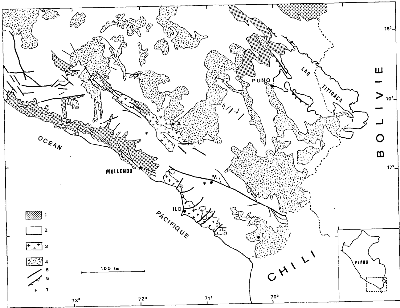
Fig. 1. — Esquisse structurale du Sud du Pérou.
