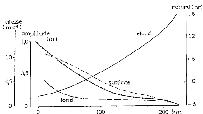
FIG. 9. — Diminution de l'amplitude (-----) et retard (—) de l'onde de marée (d'après BRUNET-MORET, 1970), et amortissement des courants de marée en surface (---) et au fond (-.-.-) (d'après LE RESTE, 1987). Delay and dampened amplitude (-----) of semi-diurnal tide along the river (from BRUNET-MORET, 1970), and decrease of tide currents, surface (---) and bottom (-.-.-) (from LE RESTE, 1987)
