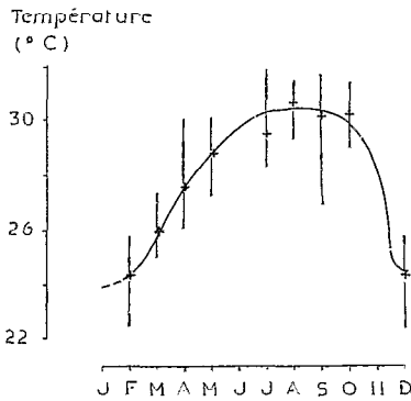
FIG. 12. — Variation annuelle de la température de l'eau. Les chiffres sont les moyennes des températures de fond mesurées lors d'une campagne, toutes stations confondues. Les barres verticales indiquent la dispersion. Annual variation of water temperature. Each monthly figure is an average of the bottom temperatures measured at all stations during the corresponding field trip
