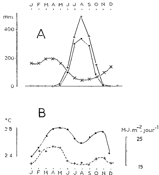
FIG. 4. — Météorologie à Ziguinchor : A : Précipitations mensuelles en période humide (1940-1960) (+) et en période sèche (1975-1985) (•), et évaporation mensuelle (1954-1959) (x...x). B : Température moyenne mesurée (1954-1959) (•—•) et rayonnement global au sol (actinométrie ASECNA) (+...+). Meteorology at Ziguinchor: A: Average monthly rainfall during a wet period (1940-1960) (+) and a dry period (1975-1985) (•), and average monthly evaporation (1954-1959) (x...x). B: Average air temperature (1954-1959) (•—•) and measured global irradiance at ground level (+...+)
