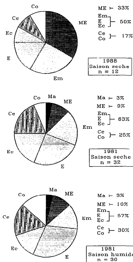
FIG. 6. — Nature des peuplements des lagunes Aghien et Potou (en saison sèche 1988, en saisons sèche et humide 1981).
