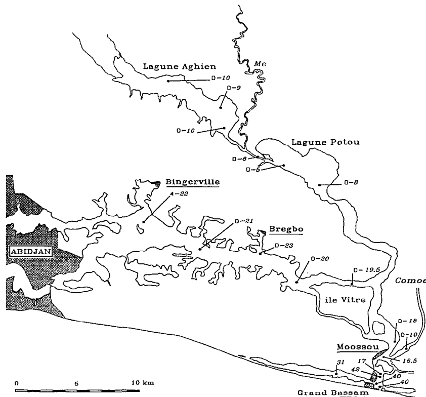
FIG. 2. — Salinités de surface relevées dans 19 stations de la partie est de la lagune en mai 1980 (première valeur) et en mai 1988 (deuxième valeur en italique)
