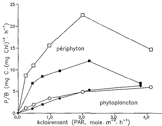
FIG. 2. — Variation du rapport P/B des communautés algales en fonction de la quantité d'énergie lumineuse (PAR) reçue.
