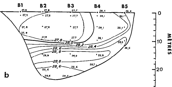
Fig. 7. — Takapoto. Valeurs mesurées et isoplèthes de S ‰ et T °C selon la coupe transversale B.
