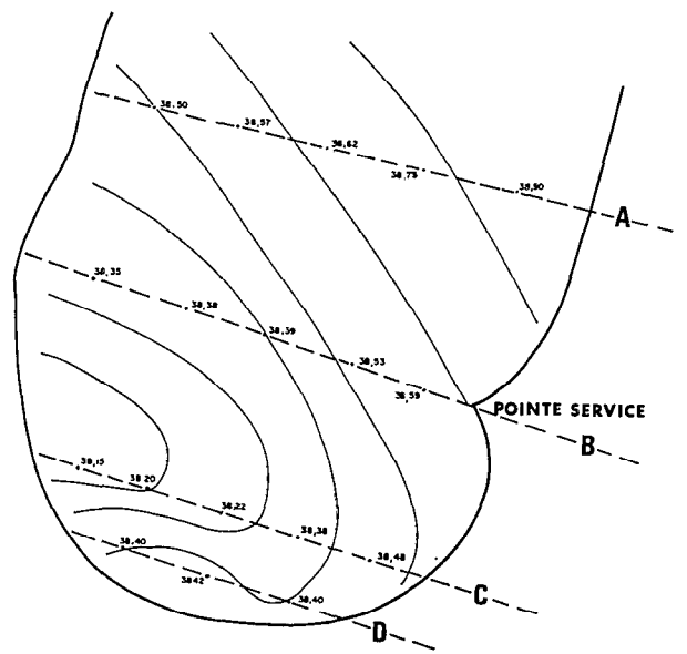
Fig. 9. — Takapoto. Distribution horizontale de la salinité de surface dans le sud du lagon.
