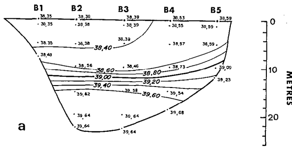
Fig. 6. — Takapoto. Valeurs mesurées et isoplèthes de S et T selon la coupe transversale A. a : Salinité ‰; b : température °C.
