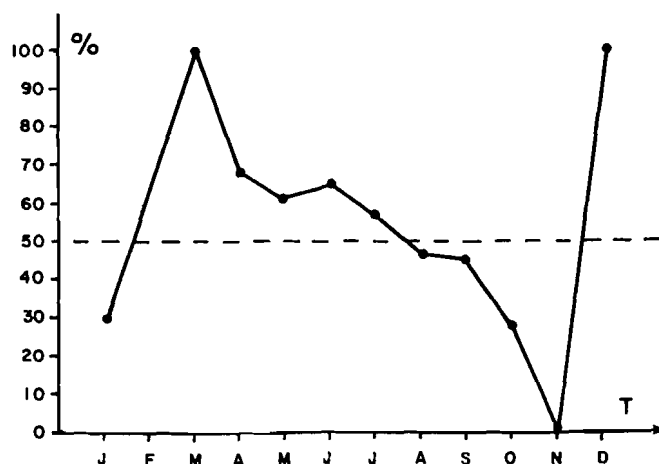
Figure 62. Evolution mensuelle de la participation des femmes à la pêche du Scylla serrata au sein du GIE "GAOU". (Source: STMMPM, 1988)
