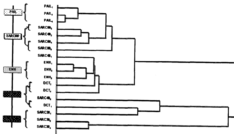
Figure 3. Classification ascendante hiérarchique des placettes étudiées selon les données de ruissellement et de pertes en terre.
