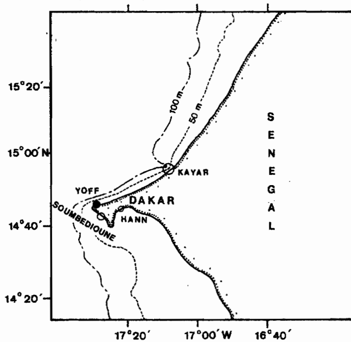
Fig.2.- Principaux centres de débarquements de la thonine au niveau de la presqu'île du Cap-Vert et station hydrologique côtière de Yoff (●)
