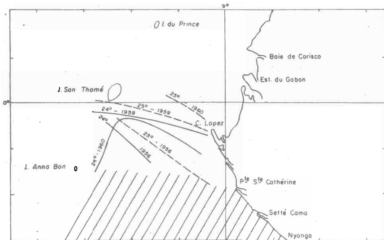
FIG. 5 - Positions des isothermes 24° et 25° en juin 1956, 1959 et 1960
