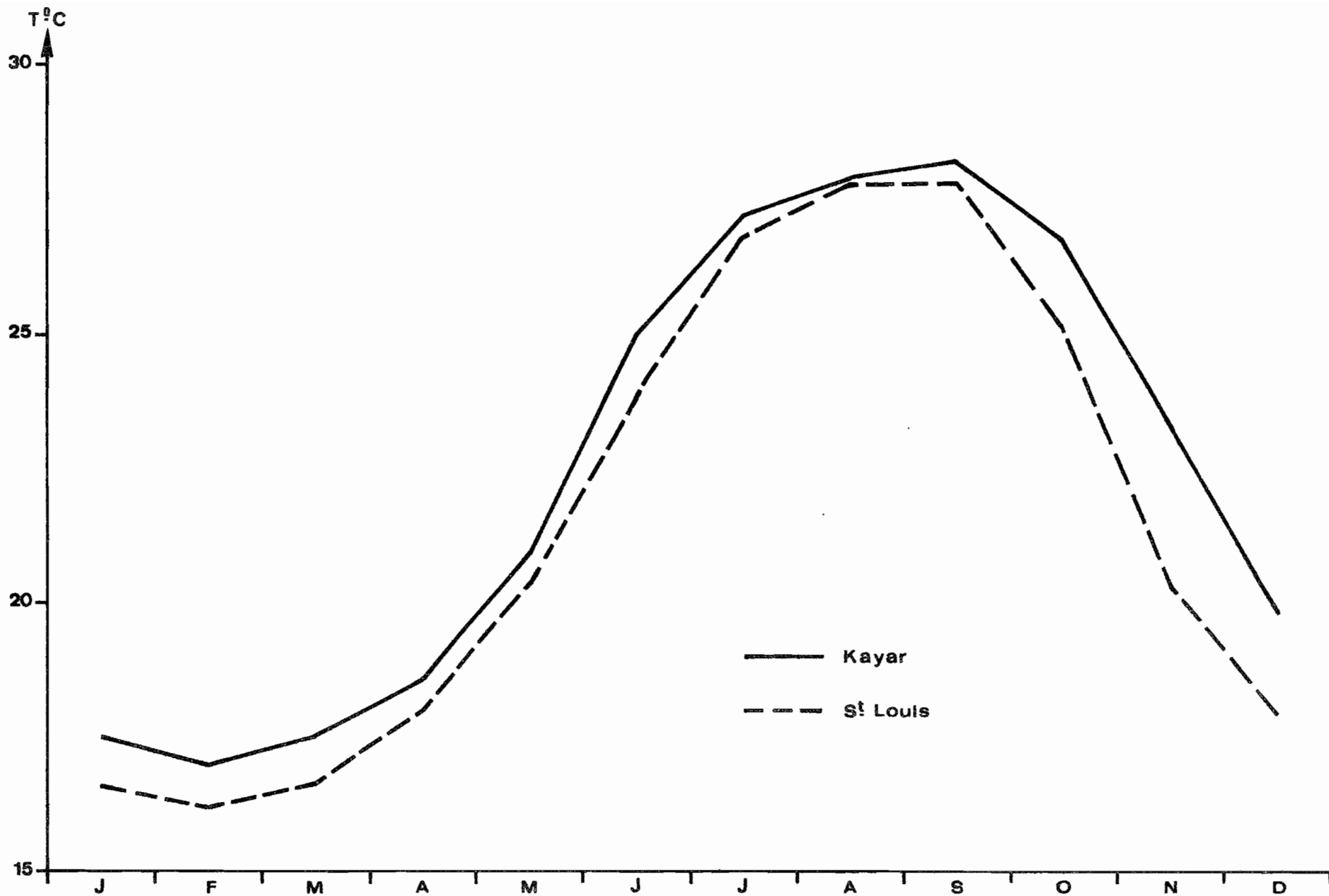
Fig.5 - TEMPERATURE ( moyenne générale ) de KAYAR . et St. LOUIS
