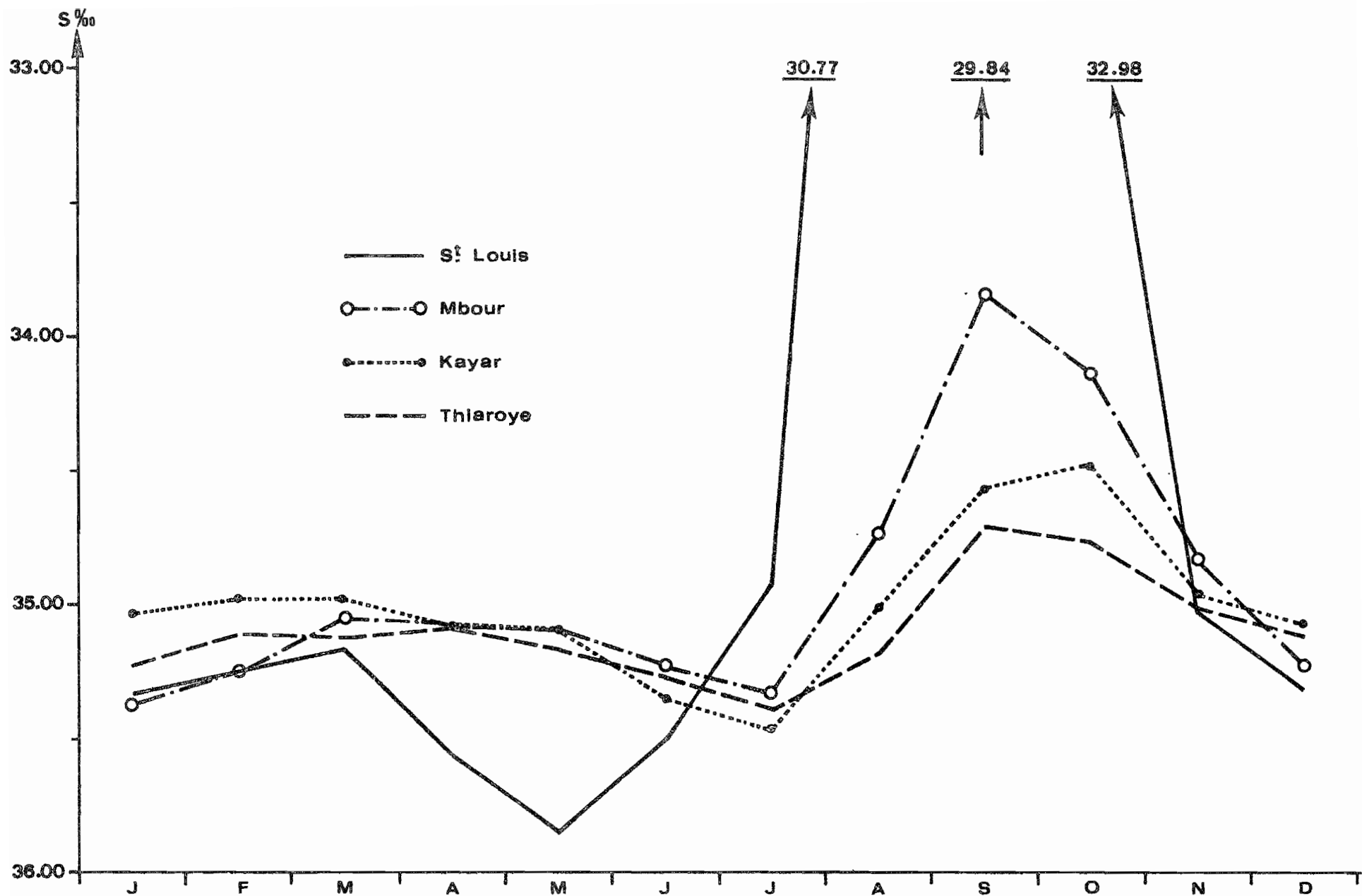
Fig.7 - SALINITE (moyenne générale) de St. LOUIS .MBOUR, KAYAR, et THIAROYE
