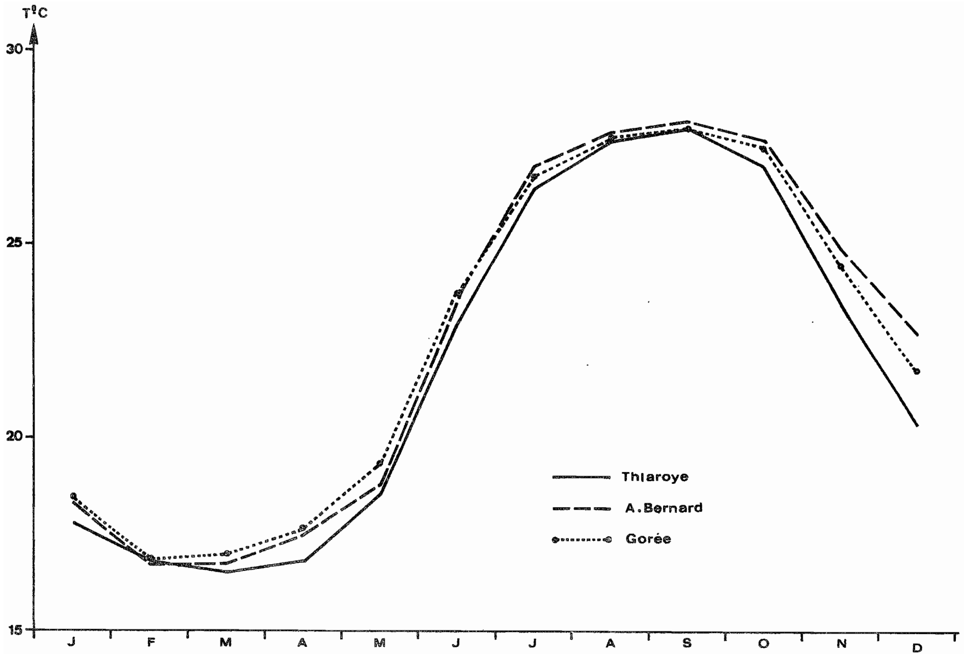
Fig. 2 - TEMPERATURE ( moyenne générale ) de THIAROYE . ANSE BERNARD, et GOREE
