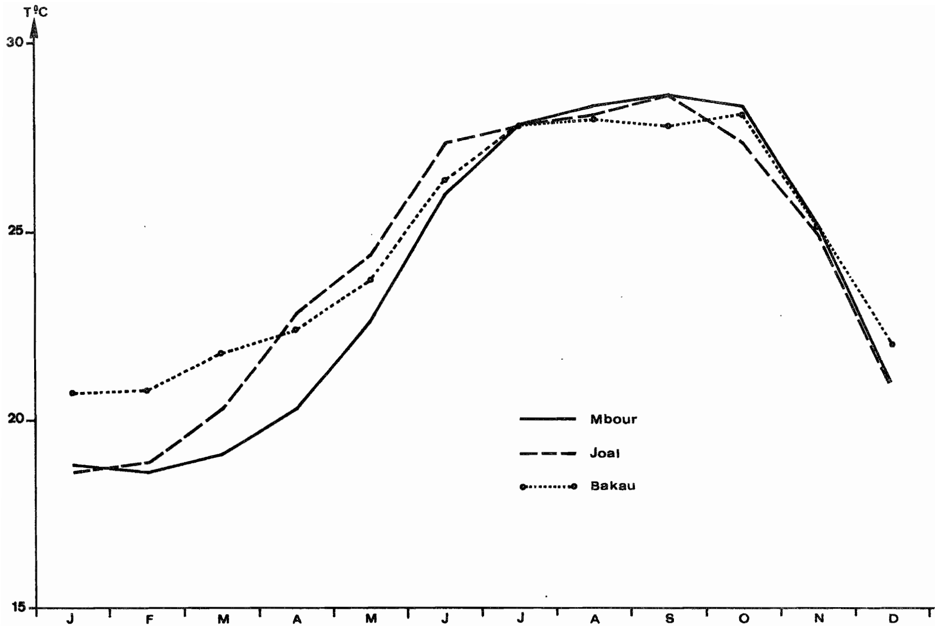
Fig. 3 - TEMPERATURE ( moyenne générale ) de MBOUR . JOAL . et BAKAU-BEACH
