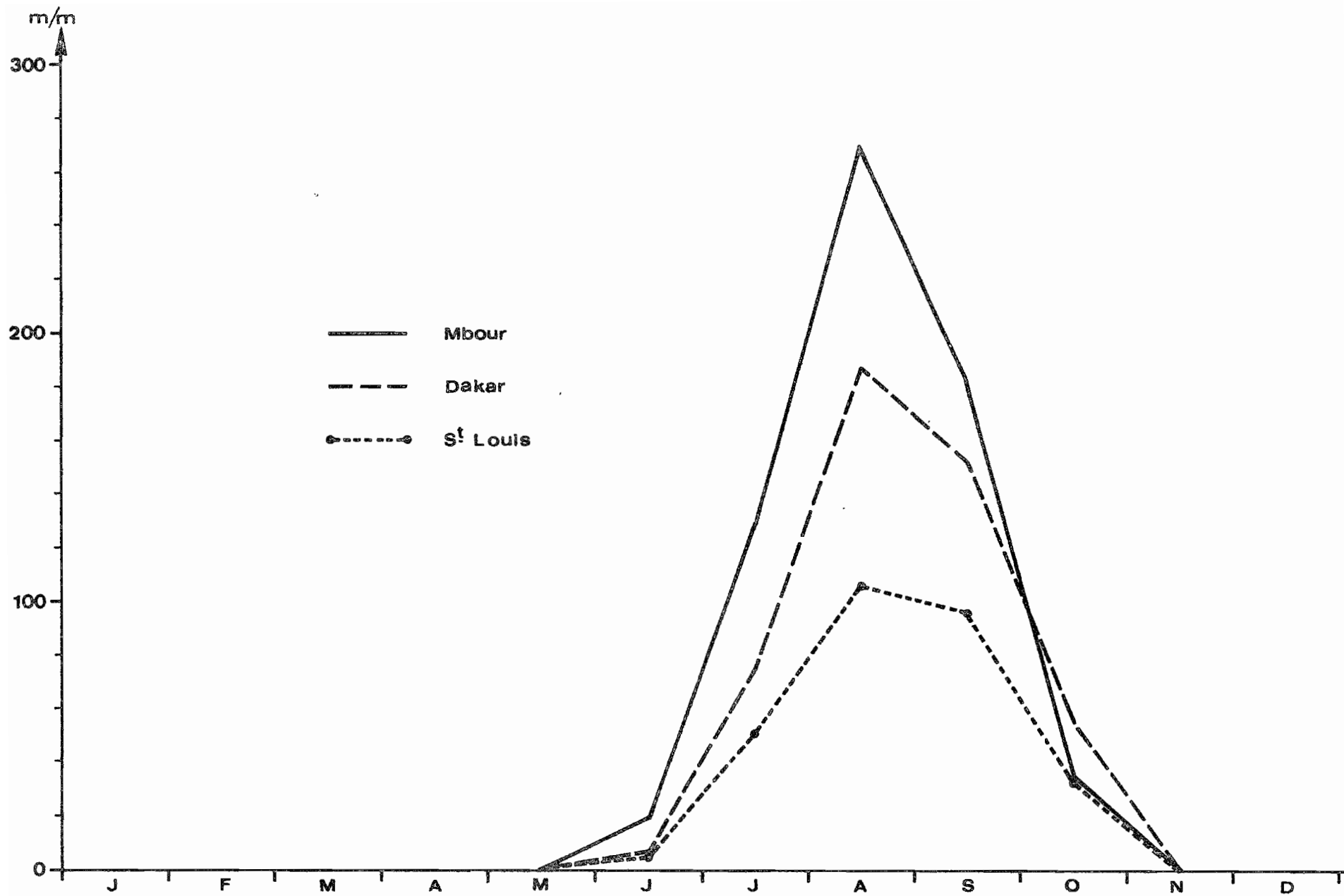
Fig. 8 - PRECIPITATIONS ( hauteur moyenne de 1960 à 1976 ) de MBOUR . DAKAR-YOFF , et St. LOUIS
