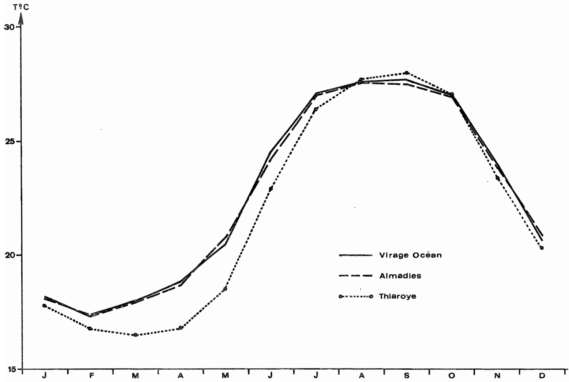
Fig. 4 - TEMPERATURE ( moyenne générale ) de VIRAGE + OCEAN . ALMADIES . et THIAROYE
