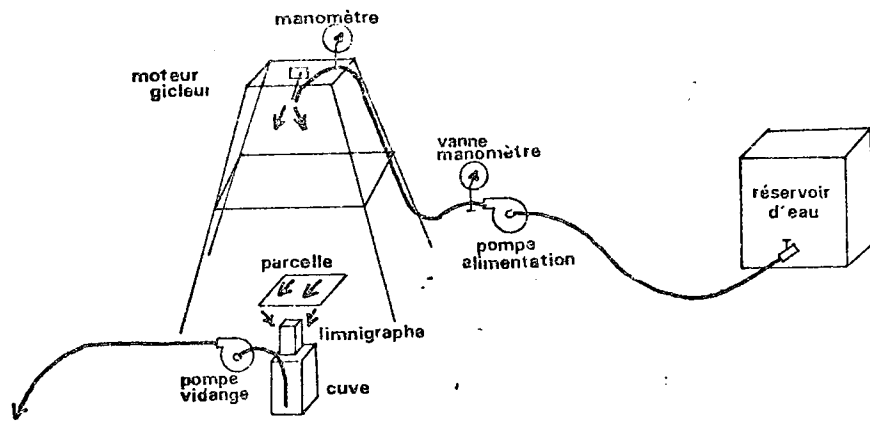
Fig. n°1 : Schéma de principe de l'infiltromètre à aspersion
