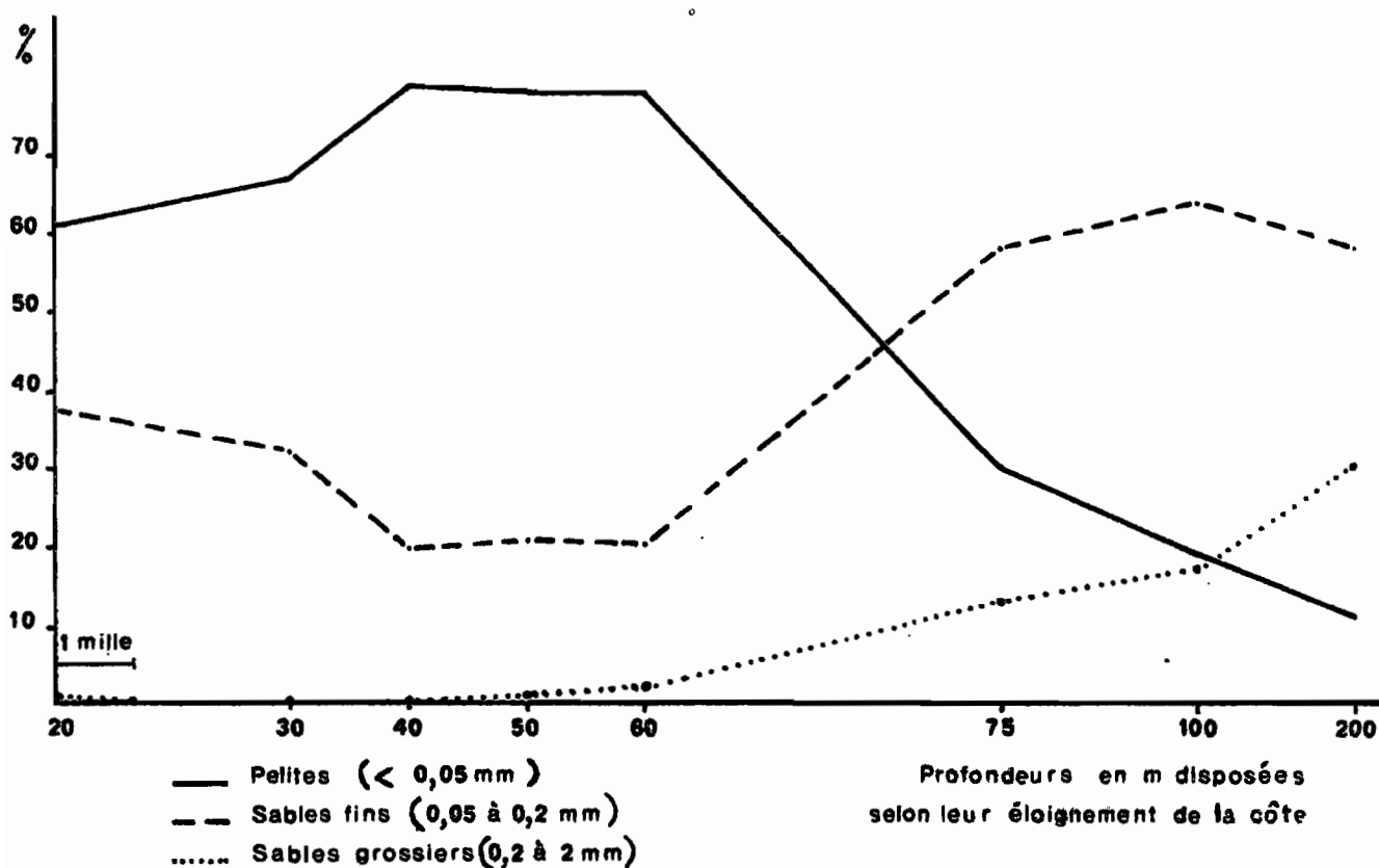
Fig.4 : Courbes de fréquence des trois fractions granulométriques rencontrées sur le fond
