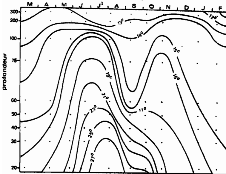
Température sur le fond fig. 1
