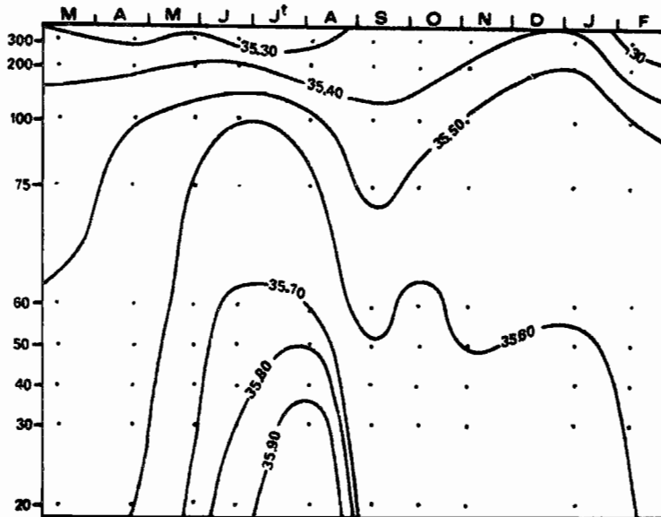
Salinité sur le fond fig. 2
