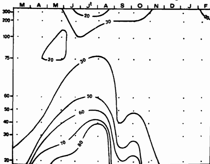
% de saturation en Oxygène dissous fig. 3
