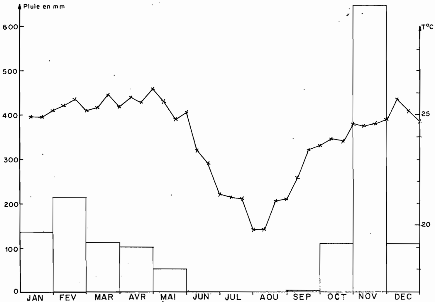
Fig. 5b - Pluviométrie au Centre O.R.S.T.O.M. 1975
