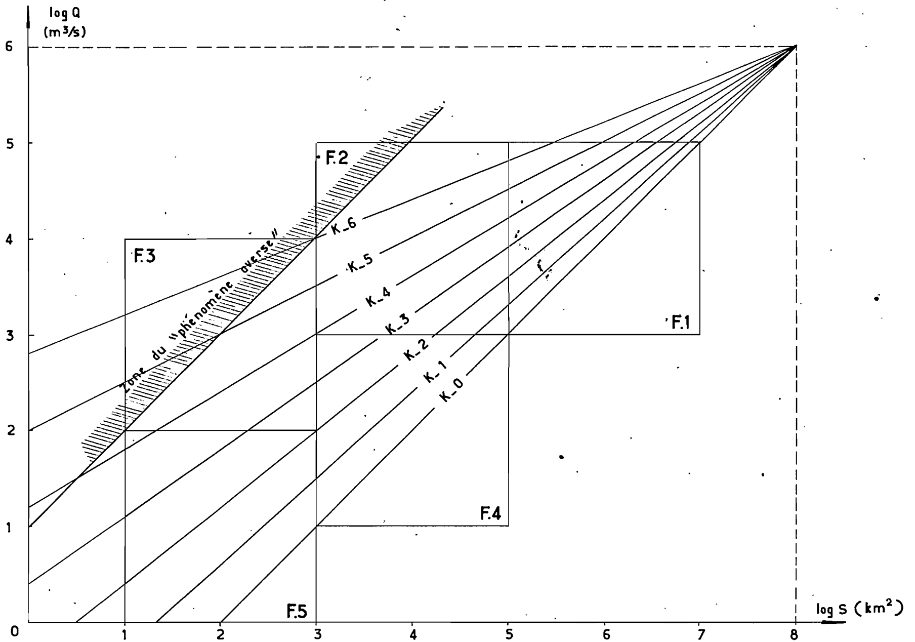
Principe du diagramme et tableau d'assemblage des 5 feuilles
