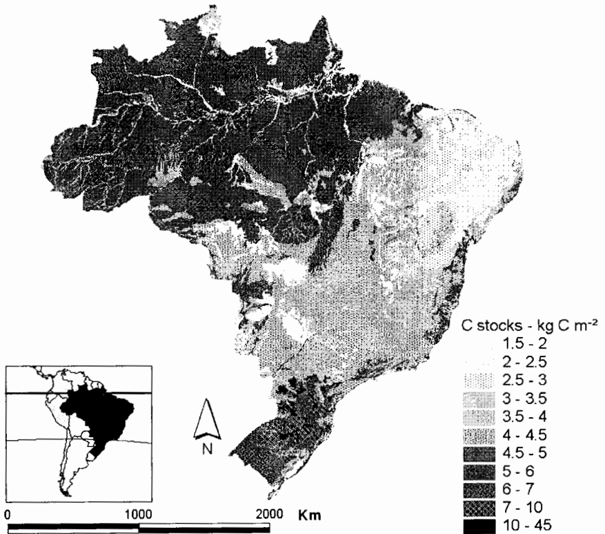
Fig. 1. Estoque de carbono nos solos (30 cm superficiais), considerando estar todo o território brasileiro sob vegetação nativa. O estoque total foi estimado em 36.400 milhões de toneladas de carbono (BERNOUX et al., 2002).
