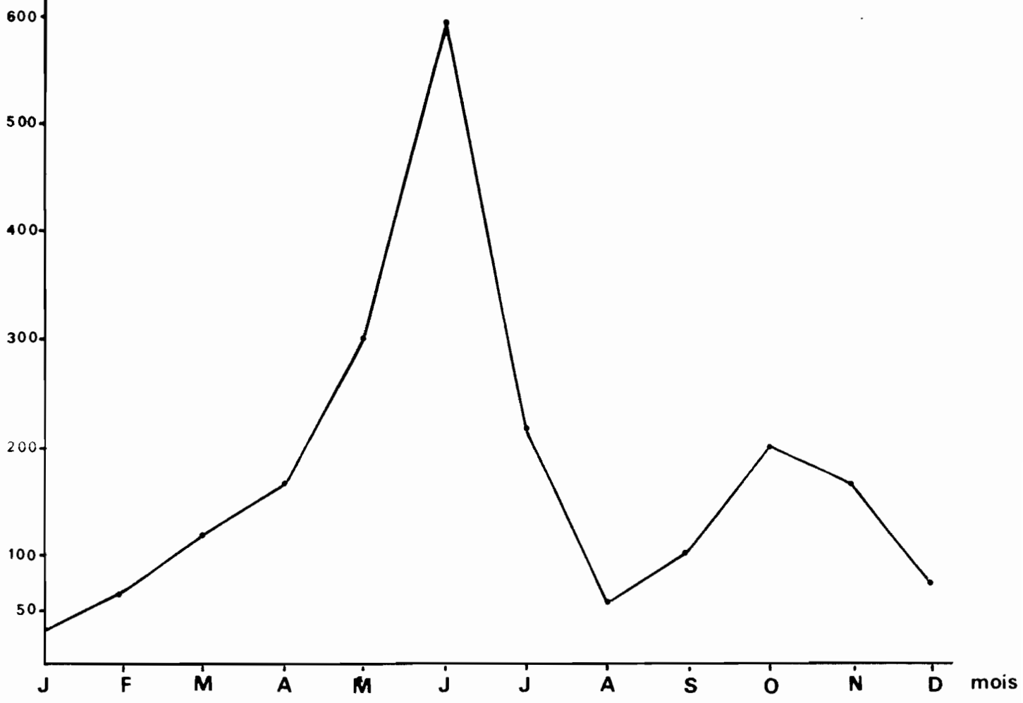
Fig : 1 Pluviométrie moyenne mensuelle de 1945 à 1980 (ASECNA)
