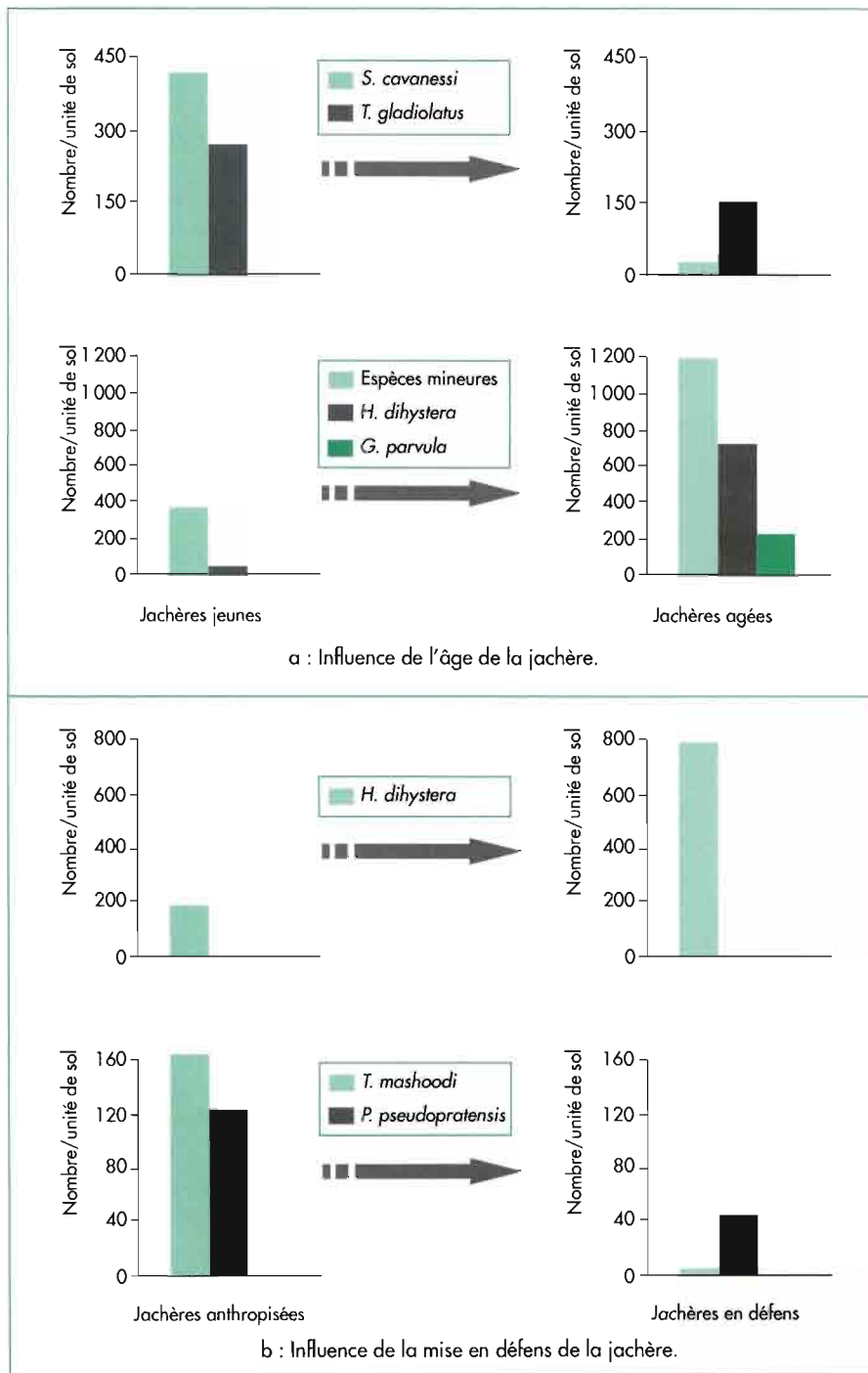
Figure 3. Récapitulation des incidences majeures de la jachère sur l'abondance de certaines espèces de nématodes, mises en évidence par l'analyse triadique. a : Influence de l'âge de la jachère. b : Influence de la mise en défens de la jachère.
