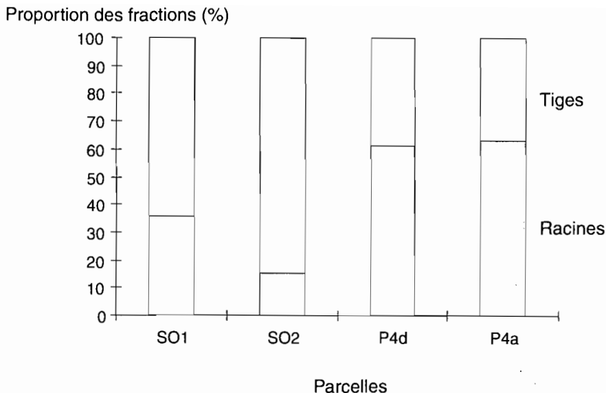
Figure 3. Proportion des fractions aérienne et souterraine.
