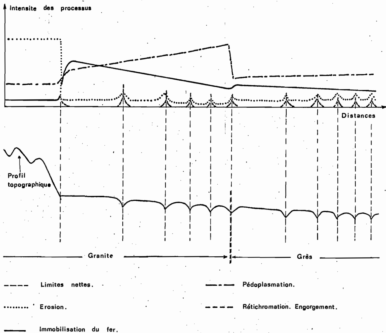
Figure 12 : Schéma des intensités relatives de certains processus pédogénétiques en zone équatoriale : limites nettes .
