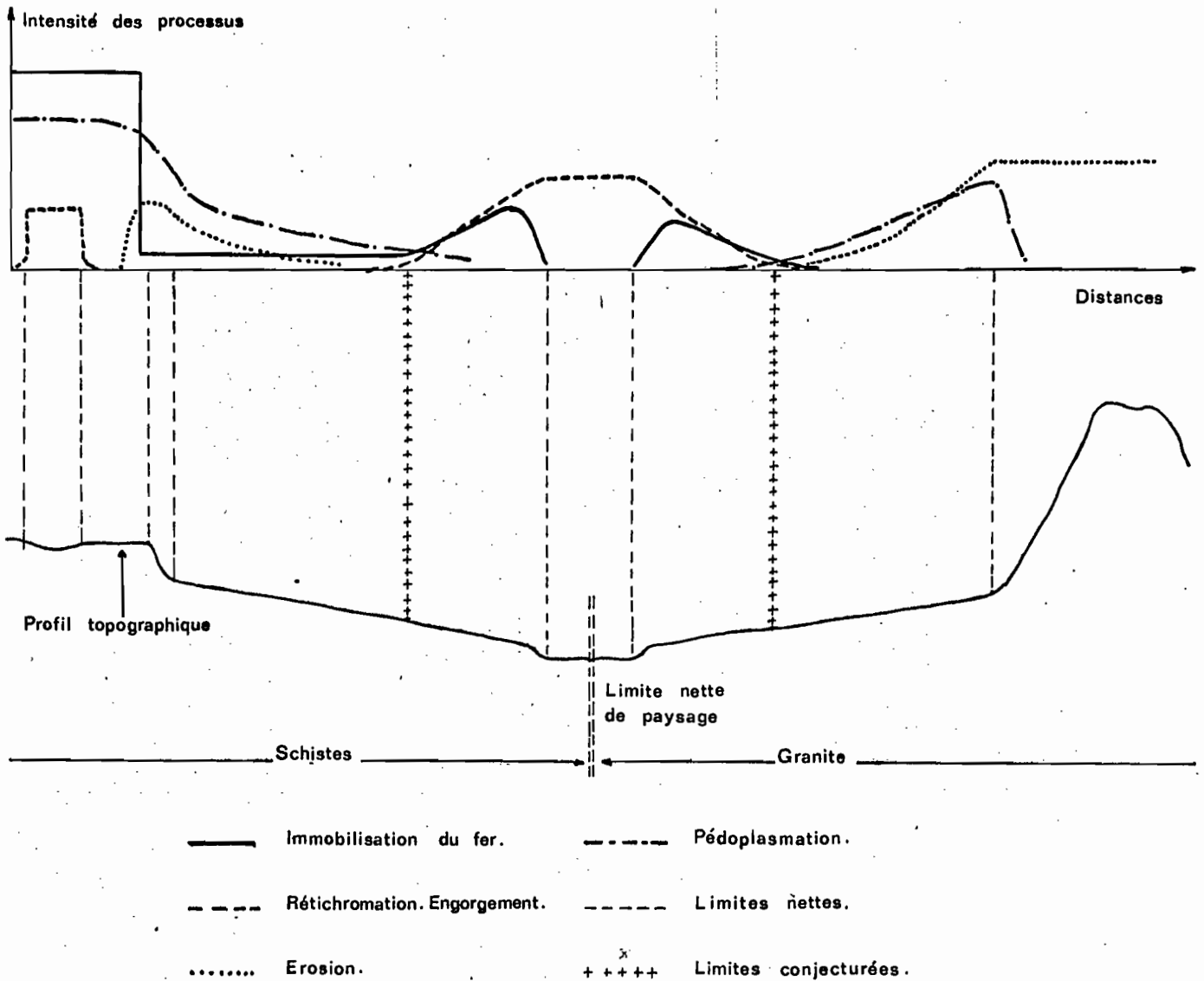
Figure 11 : Schéma des intensités relatives de certains processus pédogénétiques en zone tropicale humide, limites nettes et conjecturées.
