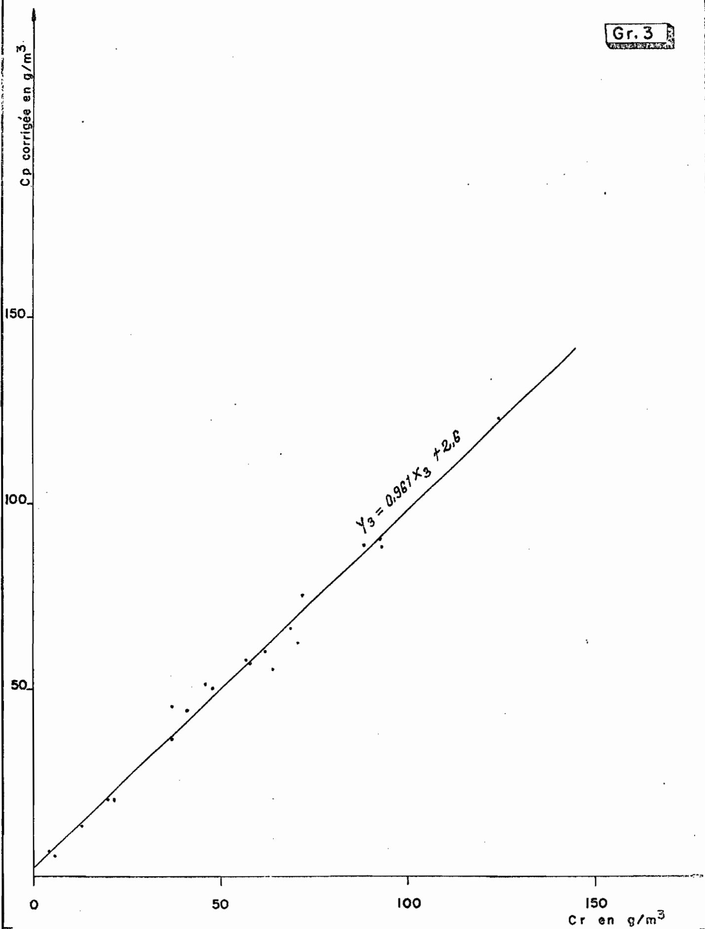
SANAGA à NACHTIGAL 1969 Correlation entre la concentration moyenne et la concentration d'un échantillon témoin
