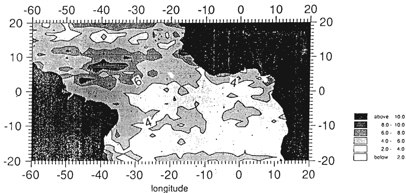
Figure 2: Variabilité saisonnière de la topographie de surface obtenue à partir des données altimétriques du satellite GEOSAT, de novembre 1986 à novembre 1987 (ARNAULT & al, 1990)
