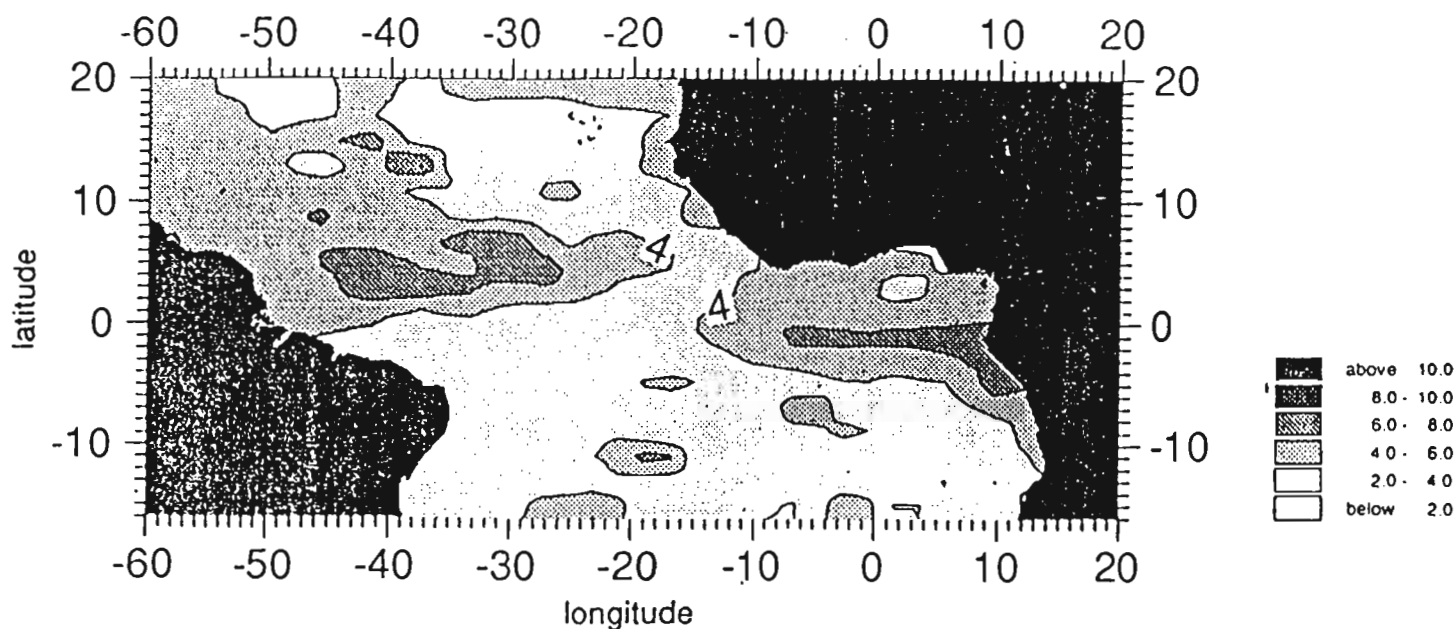
Figure 1: Variabilité saisonnière de la hauteur dynamique (5/500db) obtenue à partir de données historiques (MERLE & ARNAULT, 1984)
