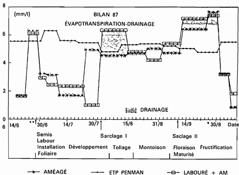
Figure 6. Evapotranspiration et drainage de l'année 1987 sur les parcelles aménagées.
