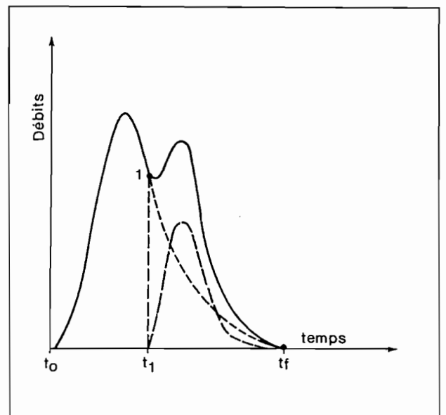
FIGURE 4 Schéma de séparation des hydrogrammes
