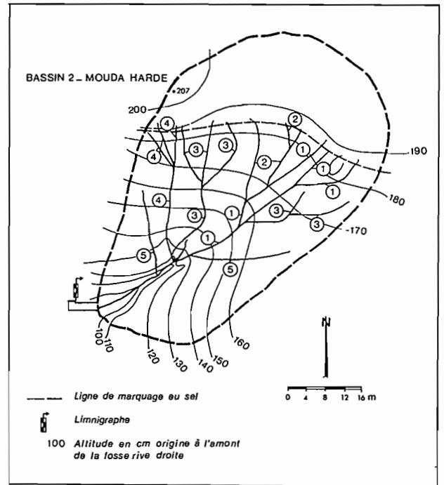
FIGURE 3 Trace des rigoles de ruissellement
