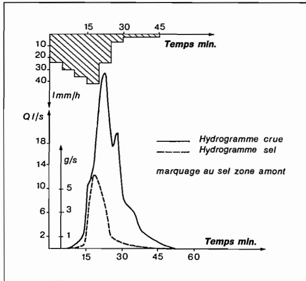
FIGURE 2 Cruie du 8 août 1986
