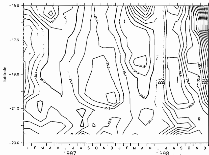
Fig 5 : Salinité de surface observée sur la ligne de navigation Nouméa-Vila-Santo de 1997 à 1998.
