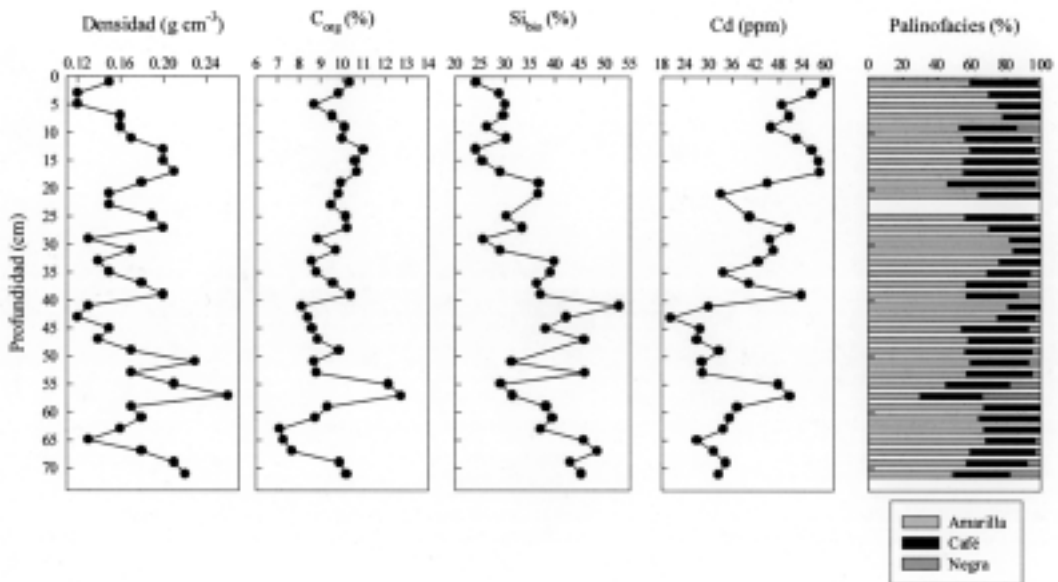
Fig. 4: Palinofacies y contenido de C_{\text{org}} , Cd y Si_{\text{bio}} en el testigo 32E. Palynofacies and content of C_{\text{org}} , Cd y Si_{\text{bio}} in the 32E core.
