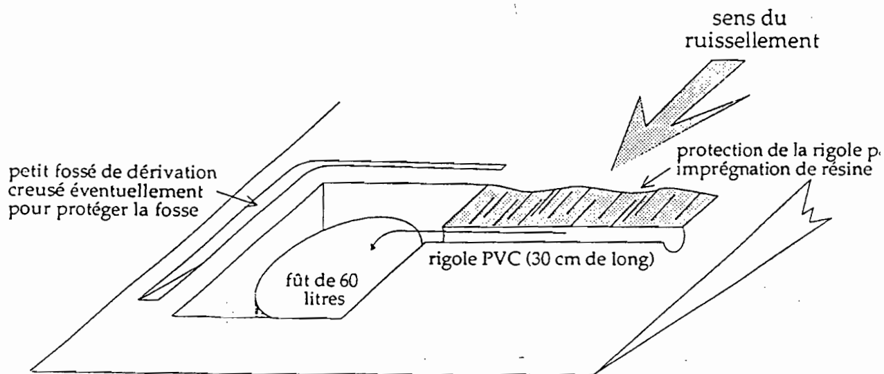
Figure 6 . Schéma d'installation d'un mini-piège.
