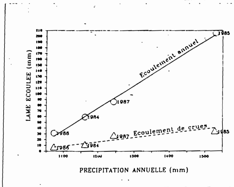
Figure 7. Bilan annuel. Relation précipitation/écoulement.
