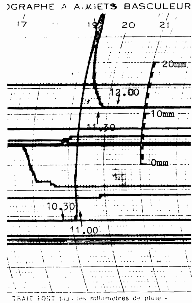
Pluviographe de PORT-BLANC
