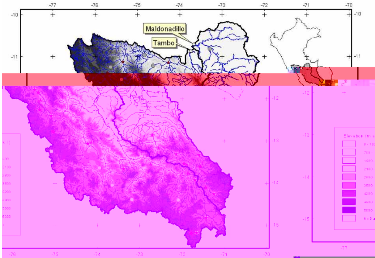
Fig. 1 Localización de la zona de estudio. Límites de las cuencas tomando como base las estaciones de descargas Tambo y Maldonadillo (o Urubamba). Círculos grises son las estaciones de lluvia, estrellas rojas son las estaciones de temperatura.
