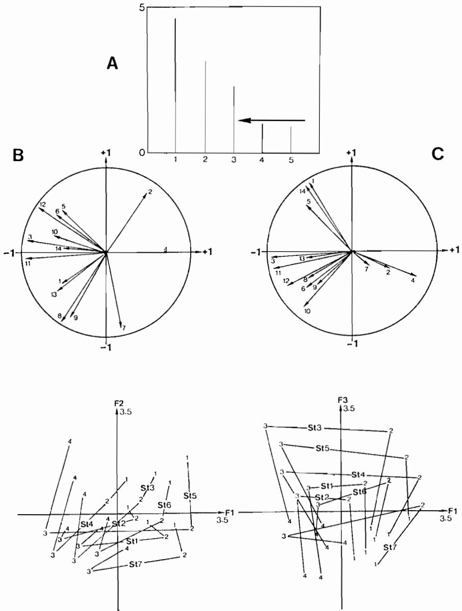
Figure 8 Analyse en composantes principales (ACP) normées du tableau des relevés physico-chimiques.
