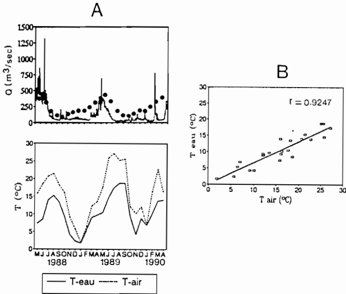
Figure 2 Variations de la température de l'eau de la Garonne et de la température de l'air en fonction du débit de la Garonne (A). Relation entre la température de l'eau et de l'air (B).
