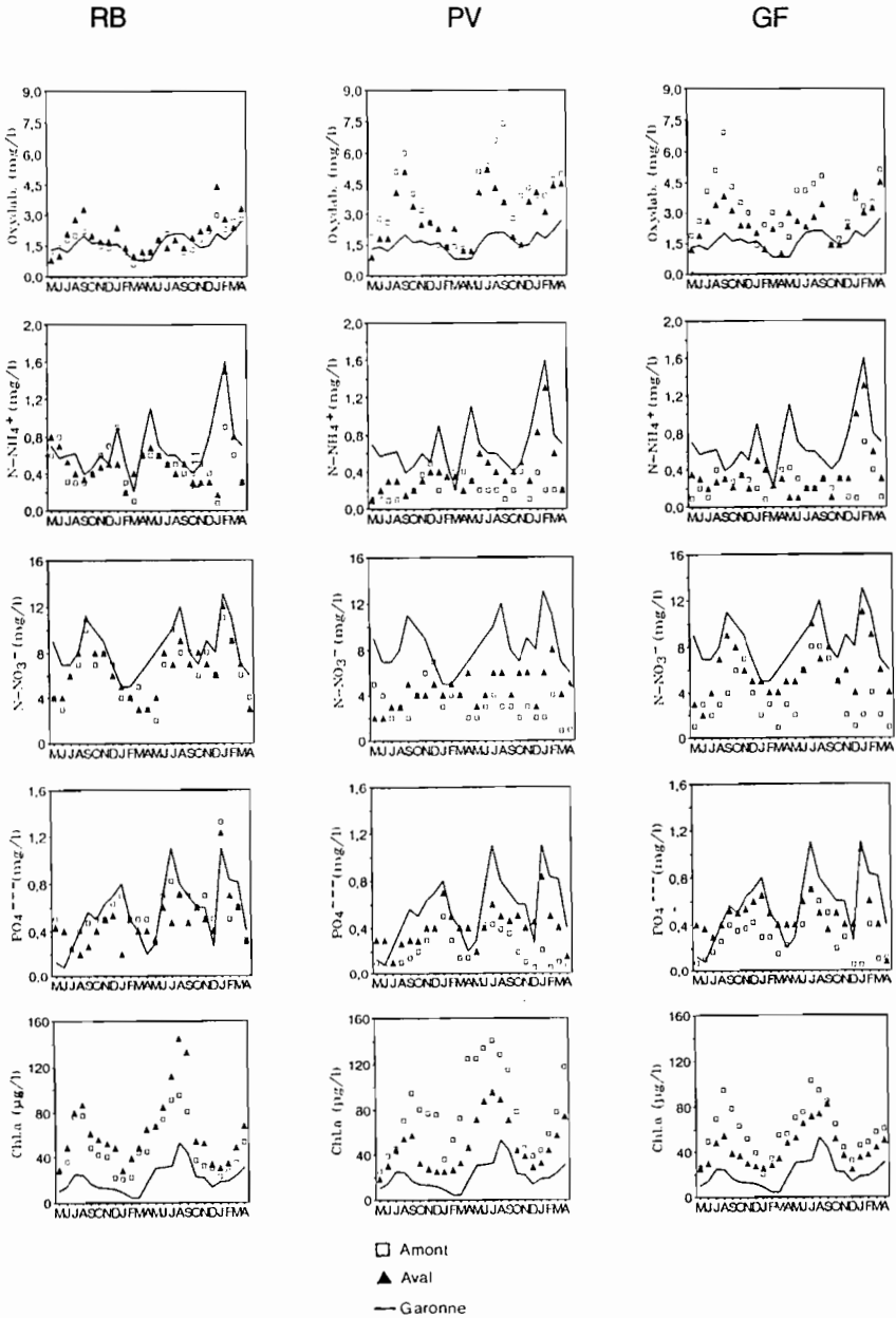
Figure 6 Evolution comparée des valeurs en oxydabilité, ammoniacque, nitrates, phosphates et chlorophylle a de trois bras morts en fonction des valeurs de la Garonne. Compared evolution of oxydability, ammonia, nitrates, orthophosphates and chlorophyll a of three ancient arms with concentrations of the river Garonne.
