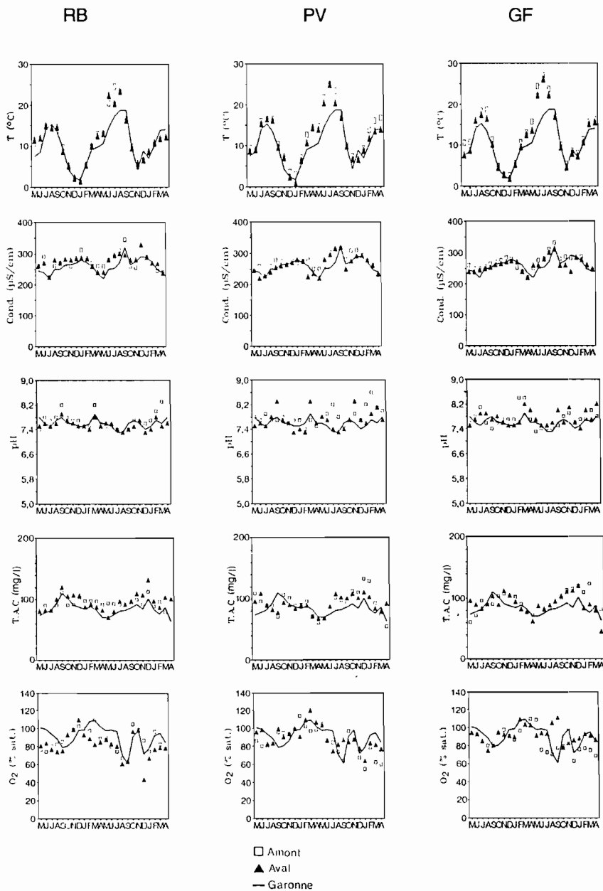
Figure 5 Evolution comparée des valeurs en température de l'eau, conductivité, pH, alcalinité total (TAC) et oxygène dissous de trois bras morts en fonction des valeurs de la Garonne.
