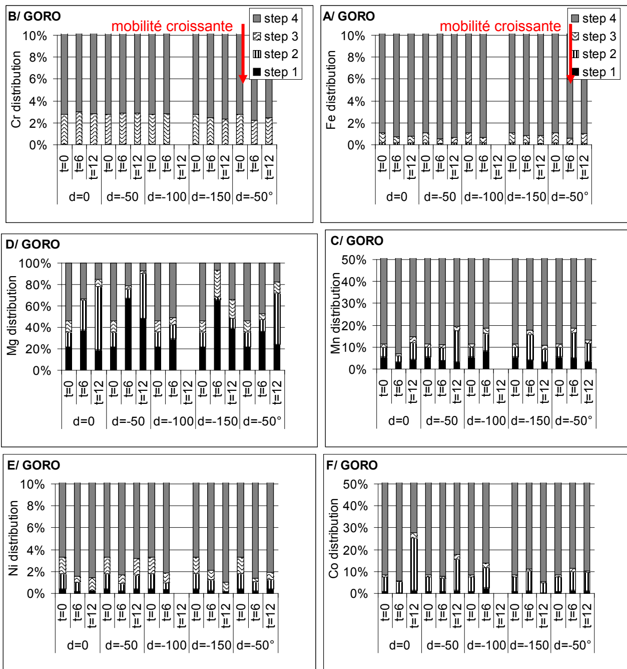
Figure 104 : Distribution des éléments métalliques dans les fractions du topsoil de Goro stocké en Andain et stocké étalé (d=-50°). Le protocole BCR isole 4 fractions les métaux : étape 1= métaux localisés dans l'eau du sol, liés aux carbonates et échangeables ; étape 2= liés aux oxydes-hydroxydes de manganèse et de fer ; étape 3=liés à la matière organique et étape 4= résiduels.
