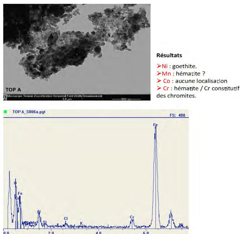
Figure 112 : Identification des minéraux par microscopie électronique à transmission et détermination de la composition des particules par sonde EDX : Particules d'hématite et de chromite dans l'horizon TOP A.
