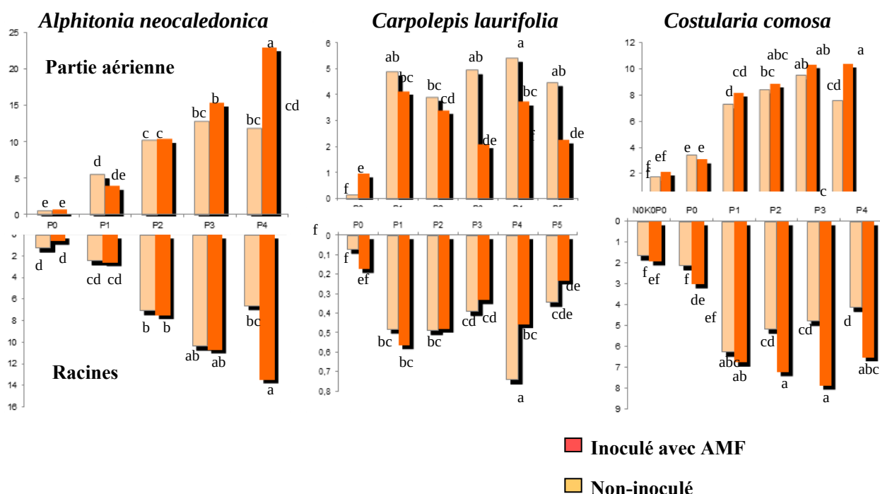
Figure 75 : Influence de la mycorhization sur la biomasse sèche (g) des plants des 3 espèces testées, après 1 an de culture en pot, sur sol fertilisé avec des doses croissantes de P.
