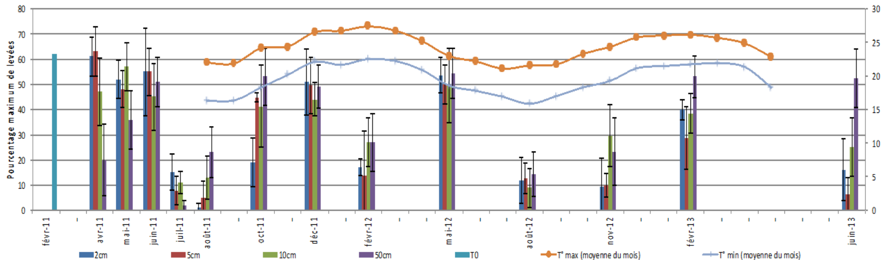
Figure 35 : Pourcentages de germination maximums (en haut) et de levées (en bas) obtenus pour les graines d' A. neocaledonica enfouies en fonction du temps à différentes profondeurs. Représentation de la température minimale et maximale entre août 2011 et mai 2013 (données VALENC).
