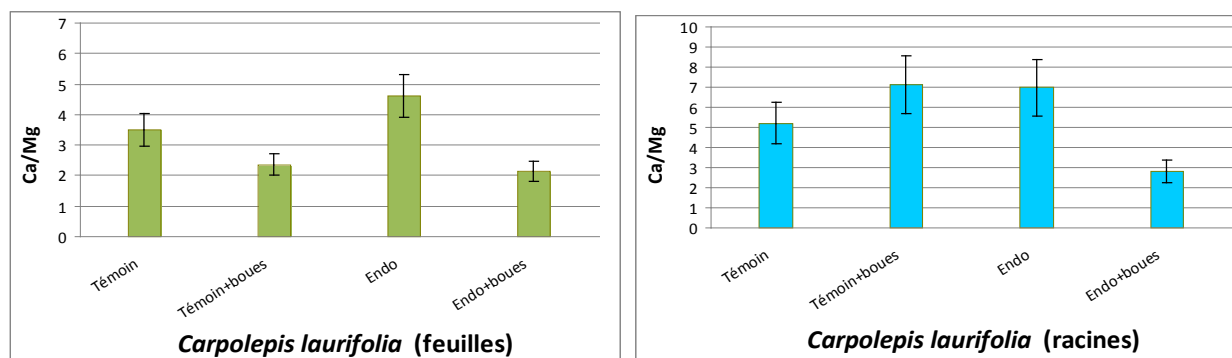
Figure 88 : Influence des boues de STEP (témoin+boues) ; des AMF (endo) et de leur combinaison (Endo+boues) sur le ratio Ca/Mg dans les différents organes de Carpolepis laurifolia , en fin d'expérience.
