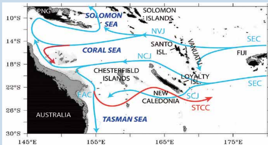
Circulation océanique autour de la Nouvelle-Calédonie. Source : CRAVATTE et al. , 2015
