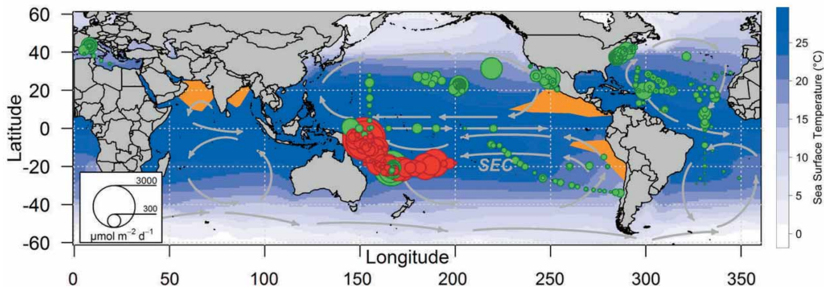
Figure 1 : Taux de fixation d'azote ( \mu\text{mol N m}^{-2} \text{ j}^{-1} ) dans le Sud-Ouest Pacifique (en rouge) comparativement aux taux mesurés dans le reste de l'océan mondial (vert). Source : BONNET et al. , 2017
