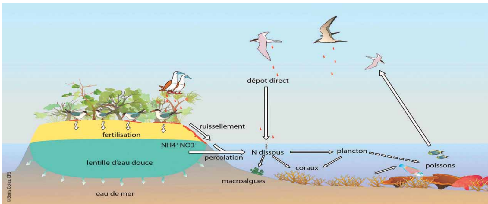
Figure 1 : Diagramme schématique de l'entrée d'azote provenant du guano dans l'écosystème corallien. Source : LORRAIN et al., 2017, modifié.
