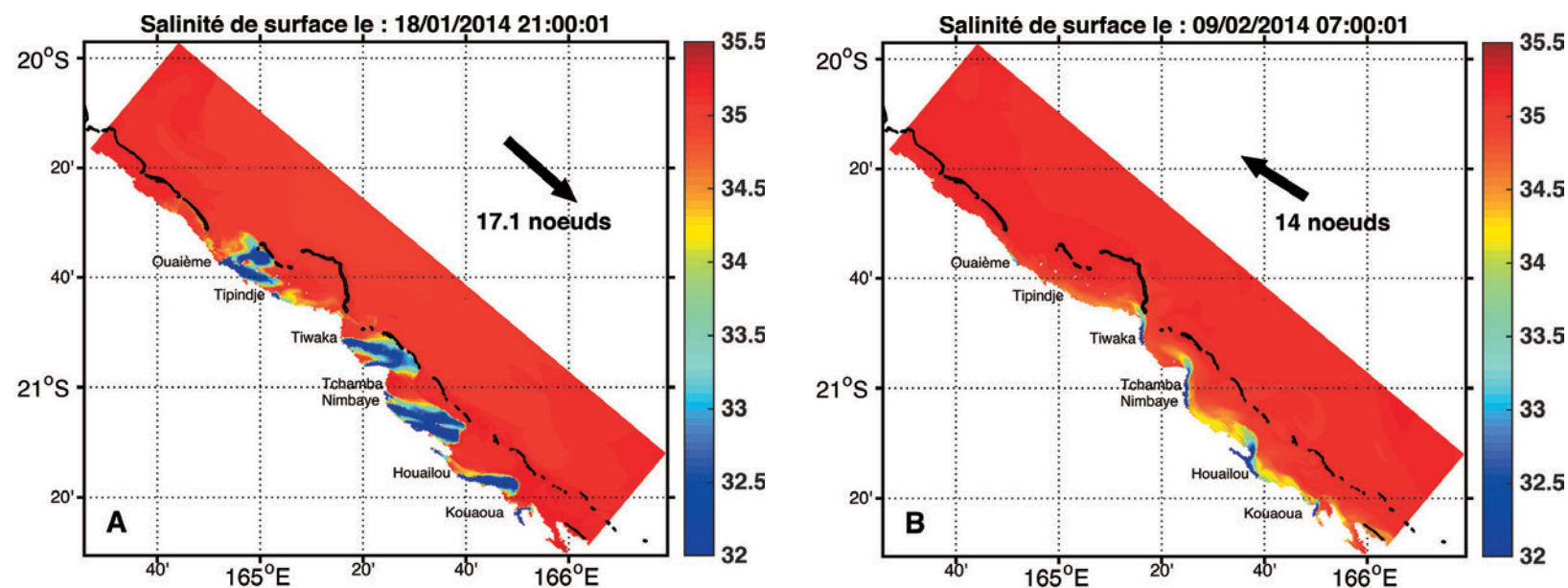
Figure 5 : Instantanés de distribution de la salinité de surface simulée par le modèle MARS3D ( http://wwwz.ifremer.fr/mars3d/ ), en unité PSU.
