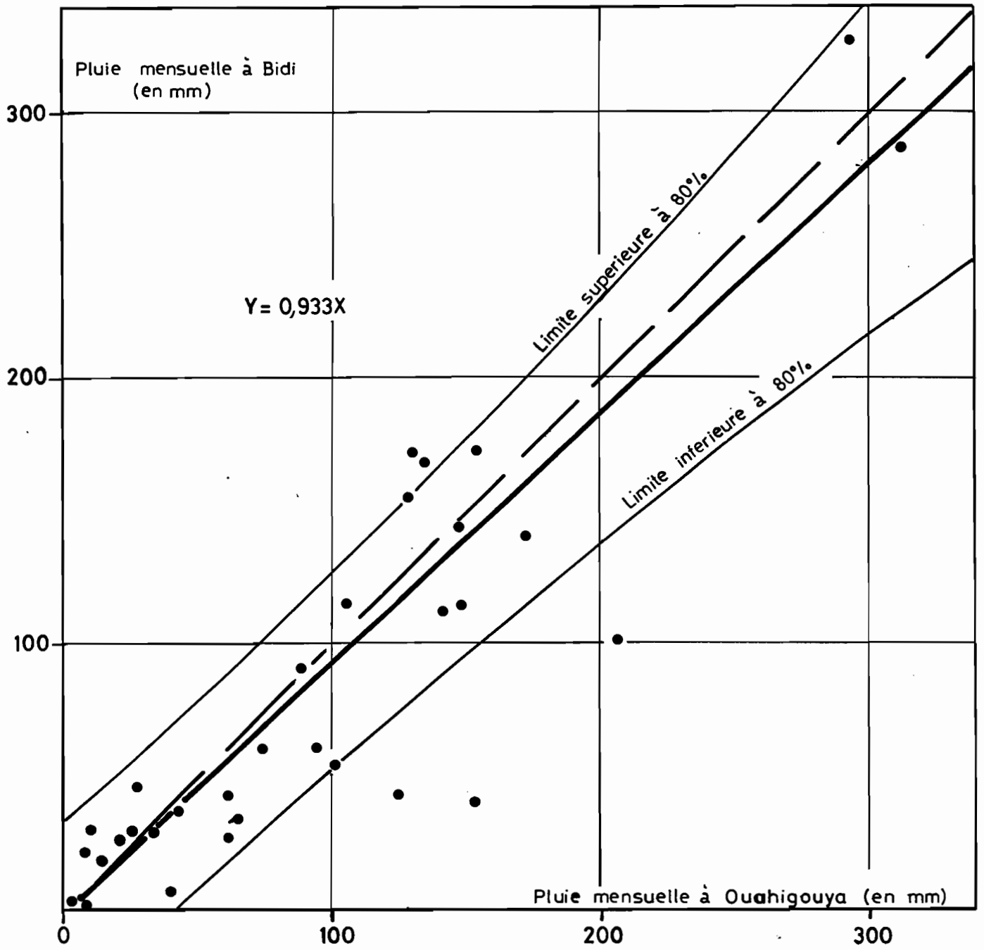
Fig. n°7 PLUIES MENSUELLES AUX POSTES DE OUAHIGOUYA ET BIDI
