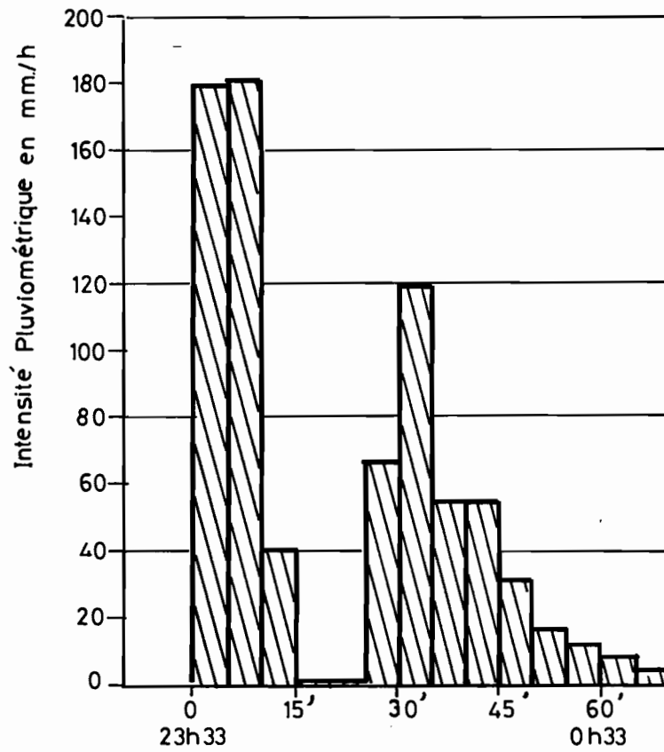
Fig. n°8 AVERSE DU 07/07 AU 08/07/92 A SAMNIWEGO
