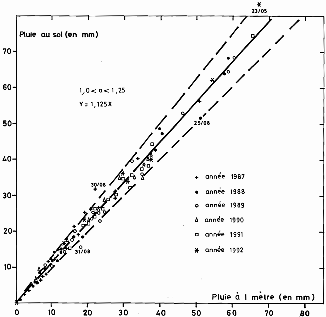
Fig. n° 13 PLUIES AU SOL ET PLUIES MESUREES/AU PLUVIOMETRE STANDARD A LA STATION DE BIDI - NAYIRI
