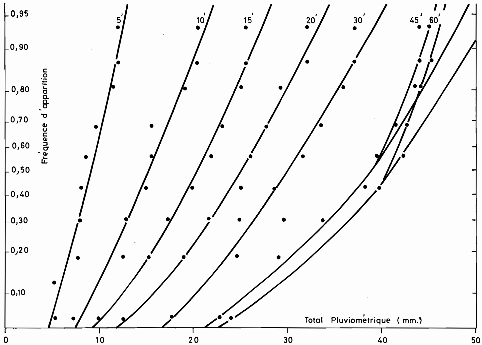
Fig. n° 17 STATISTIQUES DES PLUIES MAXIMALES AU POSTE DE BIDI-NAYIRI
