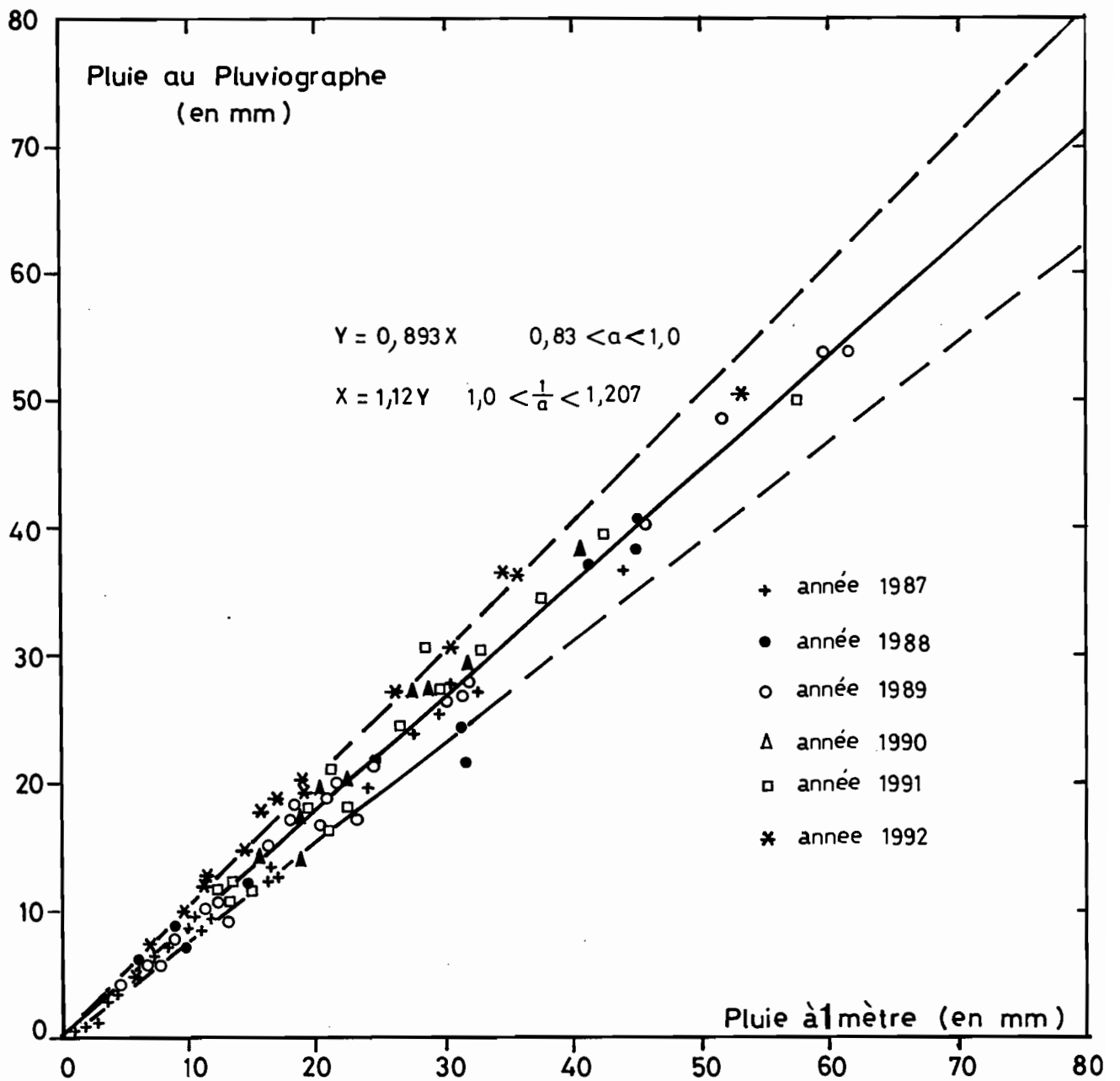
Fig n° 16 PLUIES AU PLUVIOMETRE STANDARD ET PLUIES AU PLUVIOGRAPHE A LA STATION DE SAMNIWEOGO
