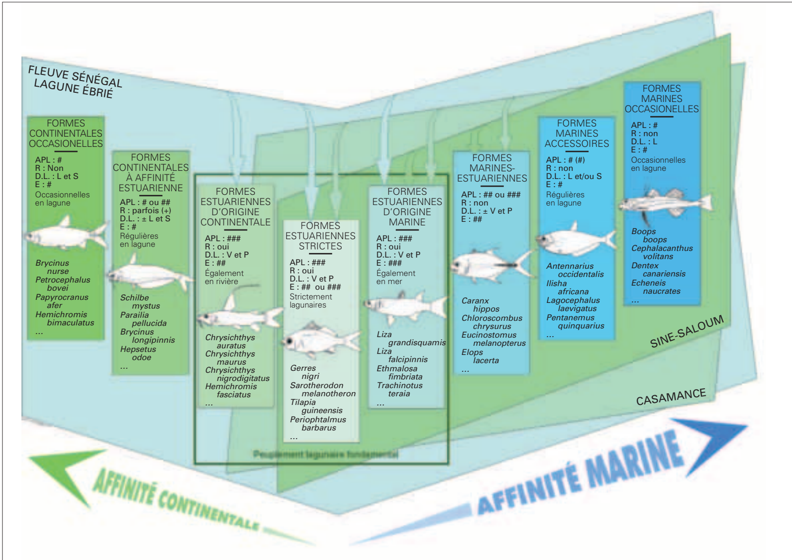
Fig. 142 – Les grandes catégories écologiques dans les peuplements de poissons des MEL d'Afrique de l'Ouest (réalisation technique : J. Vincent).
