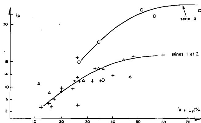
Fig. 3: Variations de I_p en fonction de la teneur du sol en éléments fins et de la nature des argiles
