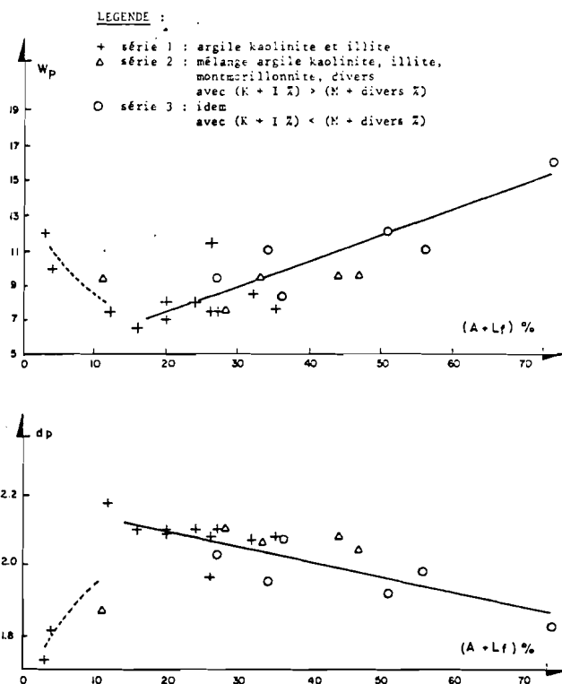
Fig. 2: Variations de w_{op} et d_p en fonction de la teneur du sol en éléments fins et de la nature des argiles
