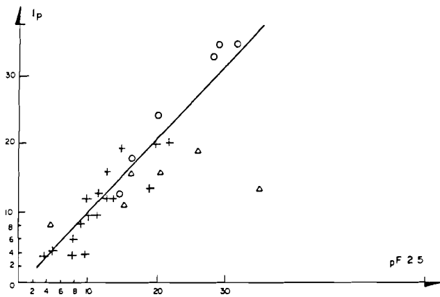
Fig. 4: Variation de I_p en fonction de la teneur en eau à pF 2,5
