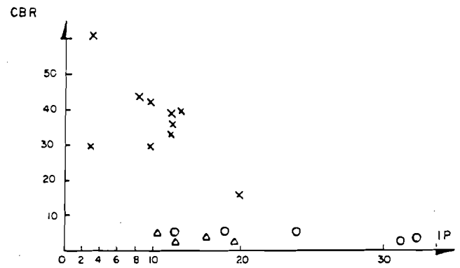
Fig. 6: Variations de CBR en fonction de I_p .
