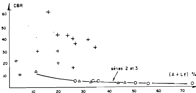
Fig. 5: Variations de CBR en fonction de la teneur du sol en éléments fins et de la nature des argiles
