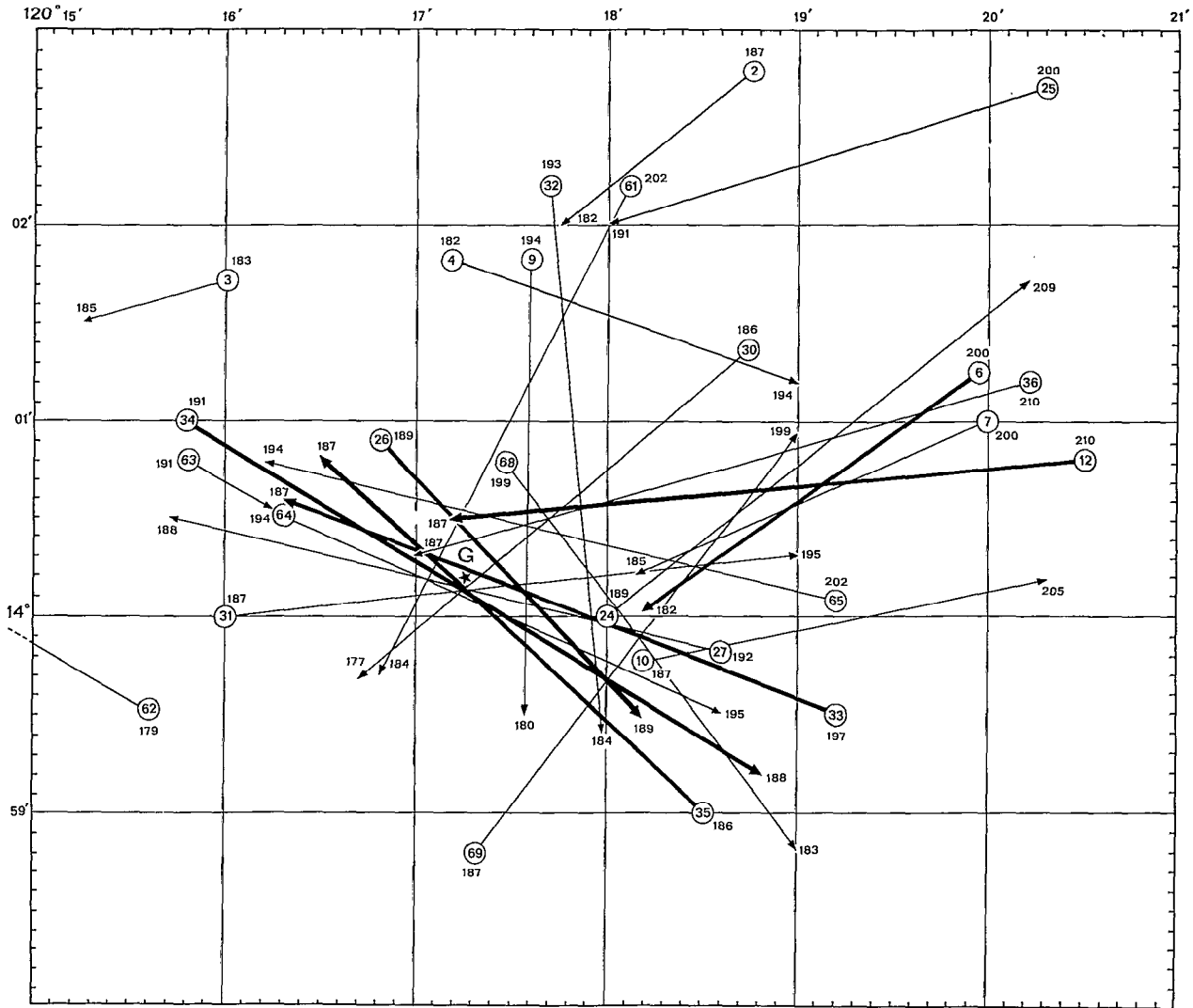
Fig. 4. — Représentation schématique des chalutages du Vauban dans la zone à Neoglyphea . L'étoile marque la station 5278 de l'« Albatross ». Voir p. 34.
