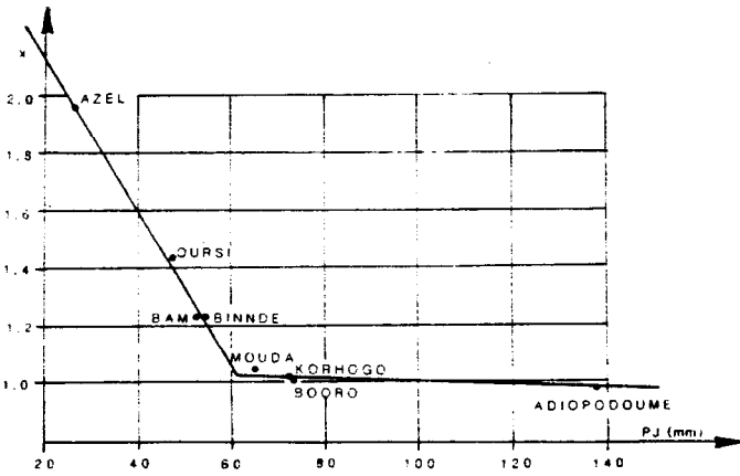
Fig-4 ECART x EN FONCTION DE LA PLUIE JOURNALIERE DE FREQUENCE ANNUELLE
