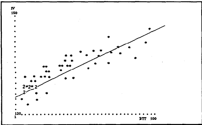
Figure 5. Régression entre l'indice de végétation (IV) et le recouvrement total de la végétation (RTT)
