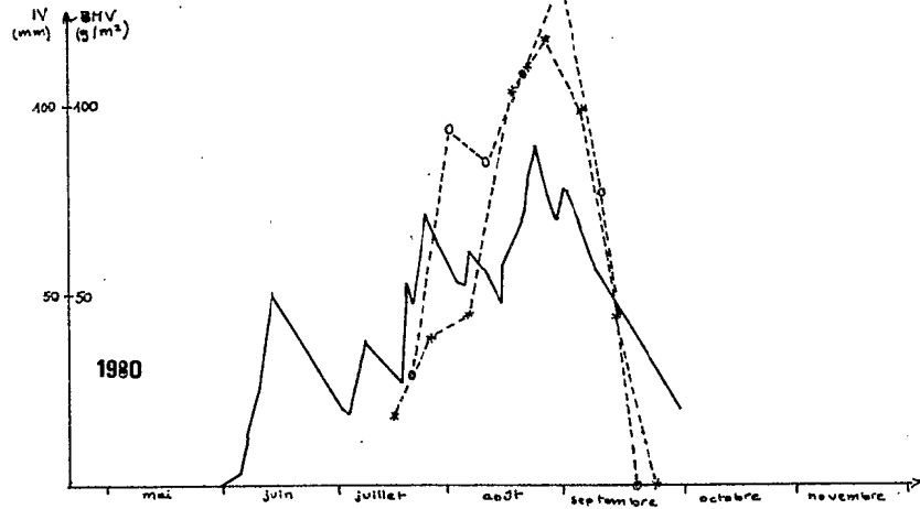
Fig. 2. — Comparaison entre la biomasse verte mesurée sur deux sites et l'indice de végétation
