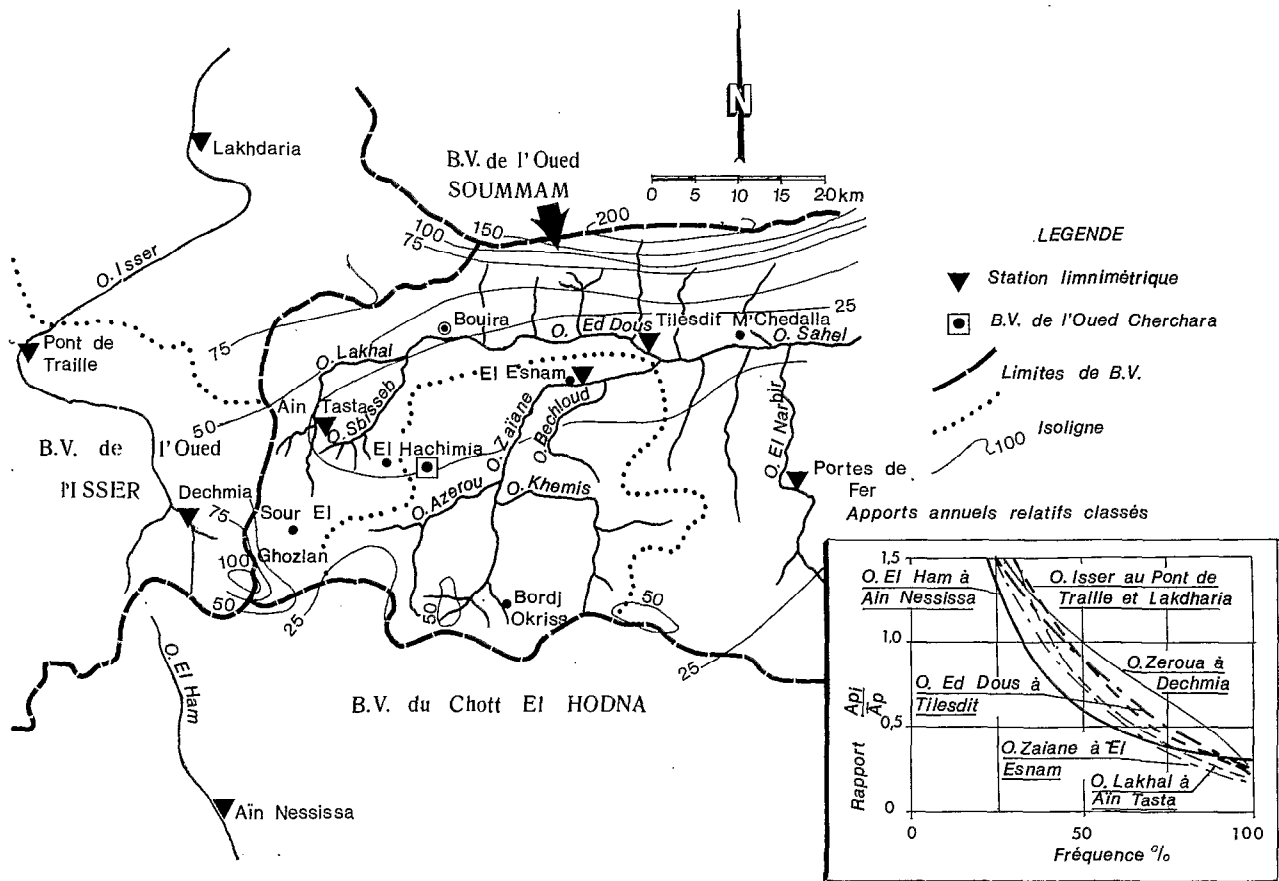
FIG. 2. — Carte des isolignes de l'écoulement annuel à 80% de fréquence de la Wilaya Bouira (en mm/an ou 10^3 \text{ m}^3/\text{km}^2 \cdot \text{an} )
