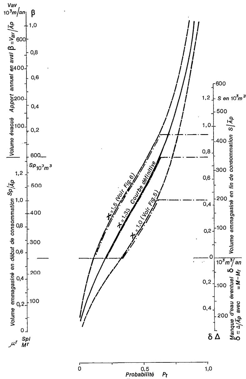
FIG. 8. — Retenue collinaire de l'Oued Cherchara — Courbe de comportement du réservoir de capacité K = 600\,000\text{ m}^3 et de rendement ( M = 250\,000\text{ m}^3/\text{an} )
