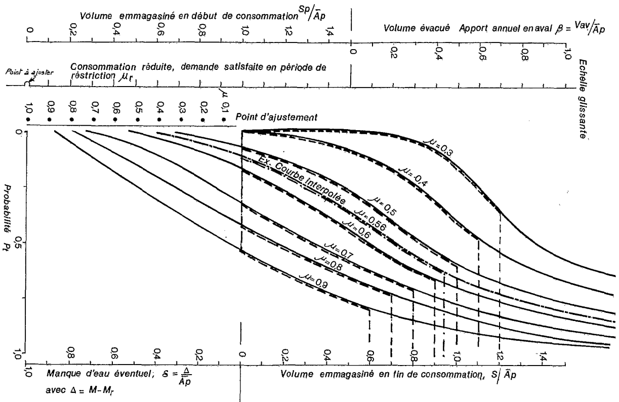
Fig. 6. — Bassin versant de l'Oued Zaïane — Abaque de comportement du réservoir pour la capacité relative \kappa = 1,5
