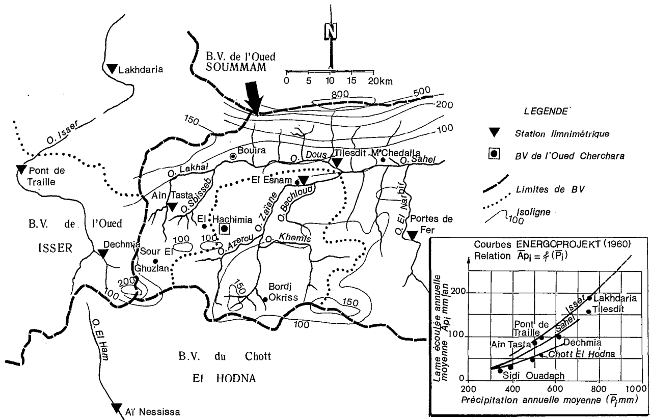
FIG. 1. — Carte isolignes de l'écoulement annuel moyen de la Wilaya Bouira (en mm/an ou 10^3 \text{ m}^3/\text{km}^2.\text{an} )
