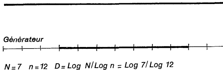
FIG. 3. — Générateur d'une poussière de Cantor de dimension \text{Log } 7 / \text{Log } 12 . A chaque étape de la génération de la poussière, chaque segment initial est divisé en n = 12 segments élémentaires. Seuls N = 7 segments élémentaires joueront, à l'étape suivante, le rôle de segment initial
