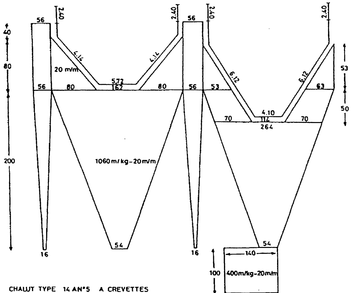
Figure 3 : Chalut à crevettes de type Le Drezen utilisé à bord des navires océanographiques de l'ORSTOM.
