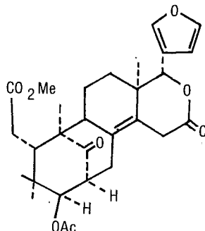
8. Fissinolide
