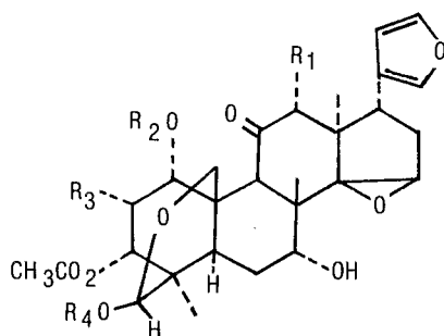
7a. Aphanastatin;
