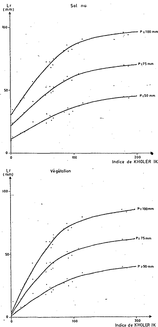
Figure 6 — Influence de l'état d'humectation initial du sol sur la hauteur de lame ruisselée.
