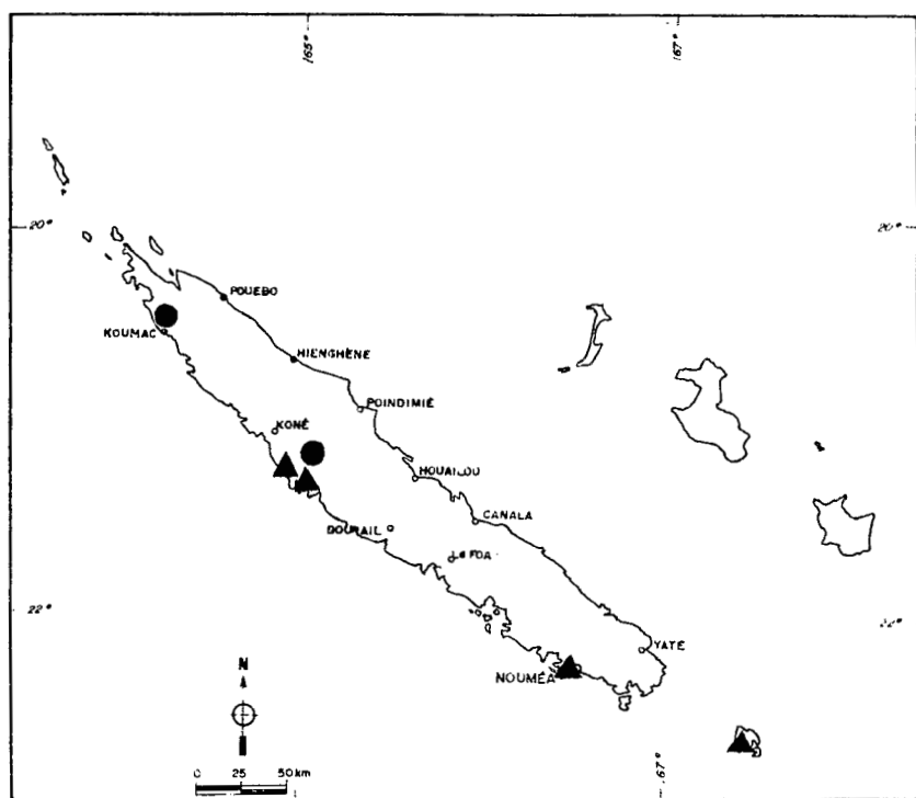
Fig. 2. — Répartition de Setaria jaffrei Morat ● et de Ancistrachne numænsis (Balansa) Blake ▲
