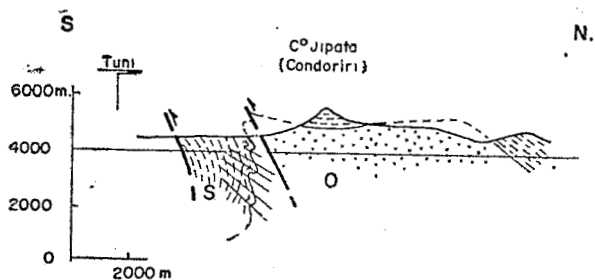
Fig 5 - Corte por la región del Tuni-Condoriri.
