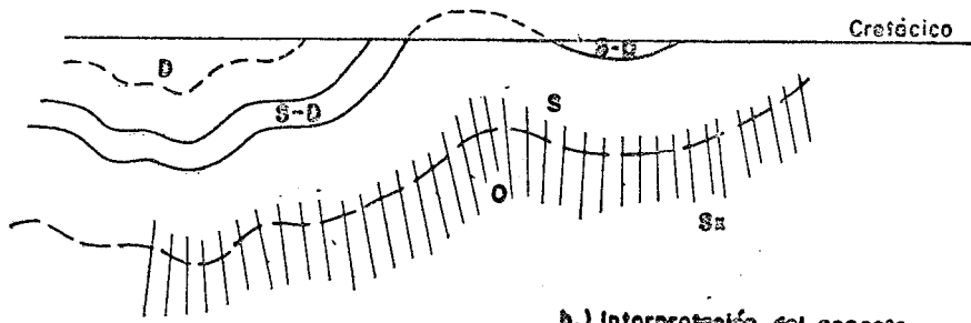
b.) Interpretación del aspecto antes de la deposición del Cretácico.
