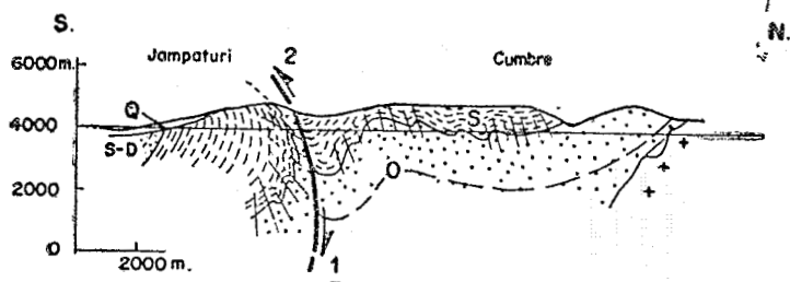
Fig. 3.- Corte estructural por Jampaturi.
