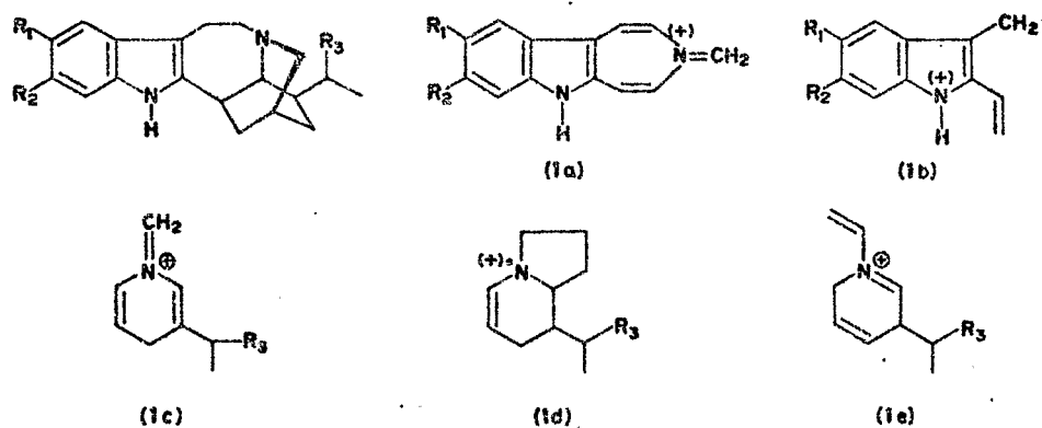
FIG. 1. SCHEMA DE FRAGMENTATION DES ALCALOÏDES DU TYPE Iboga .
