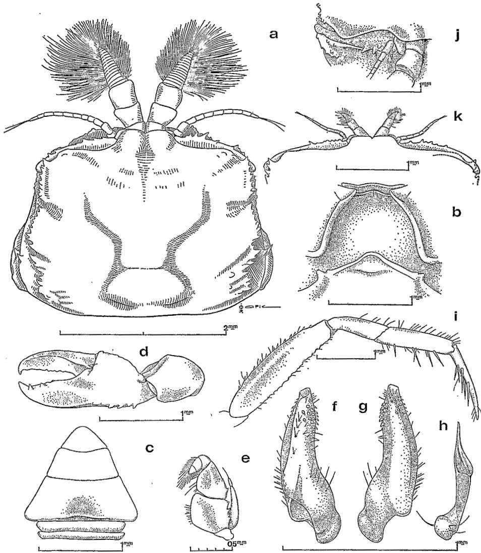
Fig. 1. Megaesthesius sagedae Rathbun, 1909. a-j, ♂ 2,3 × 3,4 mm. a, carapace; b, cavité buccale; c, abdomen; d, pince gauche; e, troisième maxillipède gauche; f, pléopode 1 gauche, face abdominale; g, pléopode 1 gauche, face sternale; h, pléopode 2 gauche, face abdominale; i, troisième périopode droit; j, région orbitaire; k, ♀ 2,6 × 3,5 mm, front, antennes et antennules.
