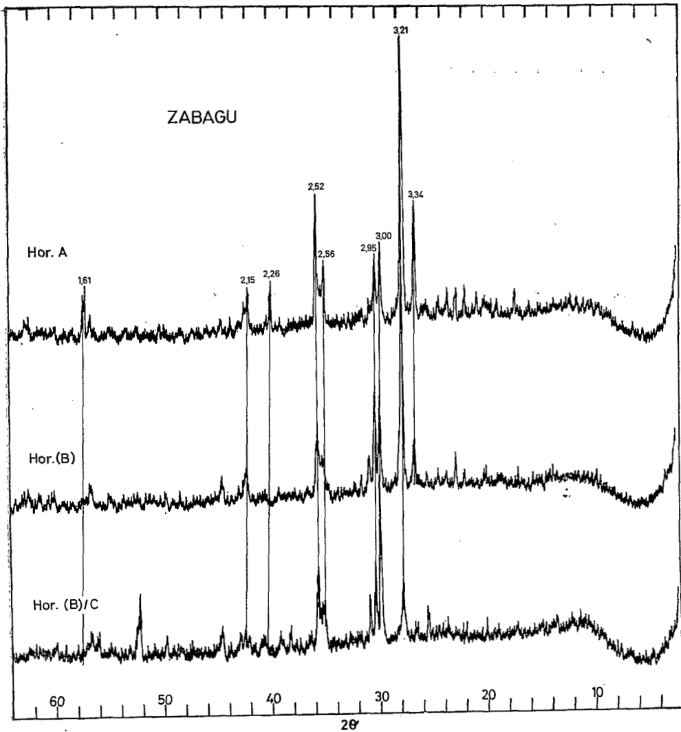
Gráfica 3.—Diagramas de difracción de rayos X, perfil «Zabagu» (método de Debye-Sherrer).
