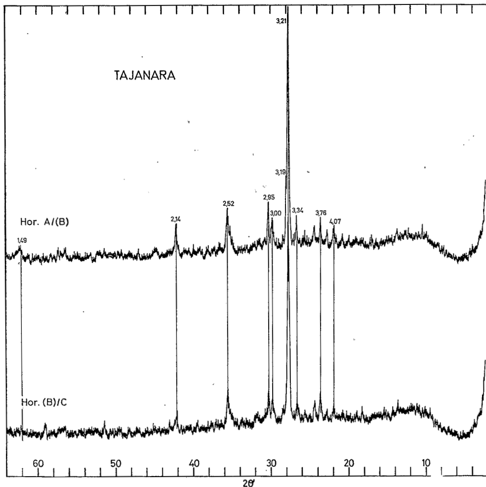
Gráfica 4.—Diagramas de difracción de rayos X, perfil «Tajamara» (método de Debye-Sherrer).
