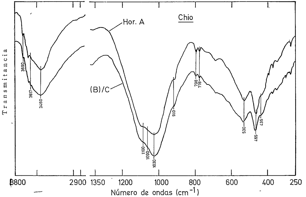
Gráfica 6.—Espectros de absorción infrarroja, entre 3.900 - 200 \text{cm}^{-1} , perfil «Chio».
