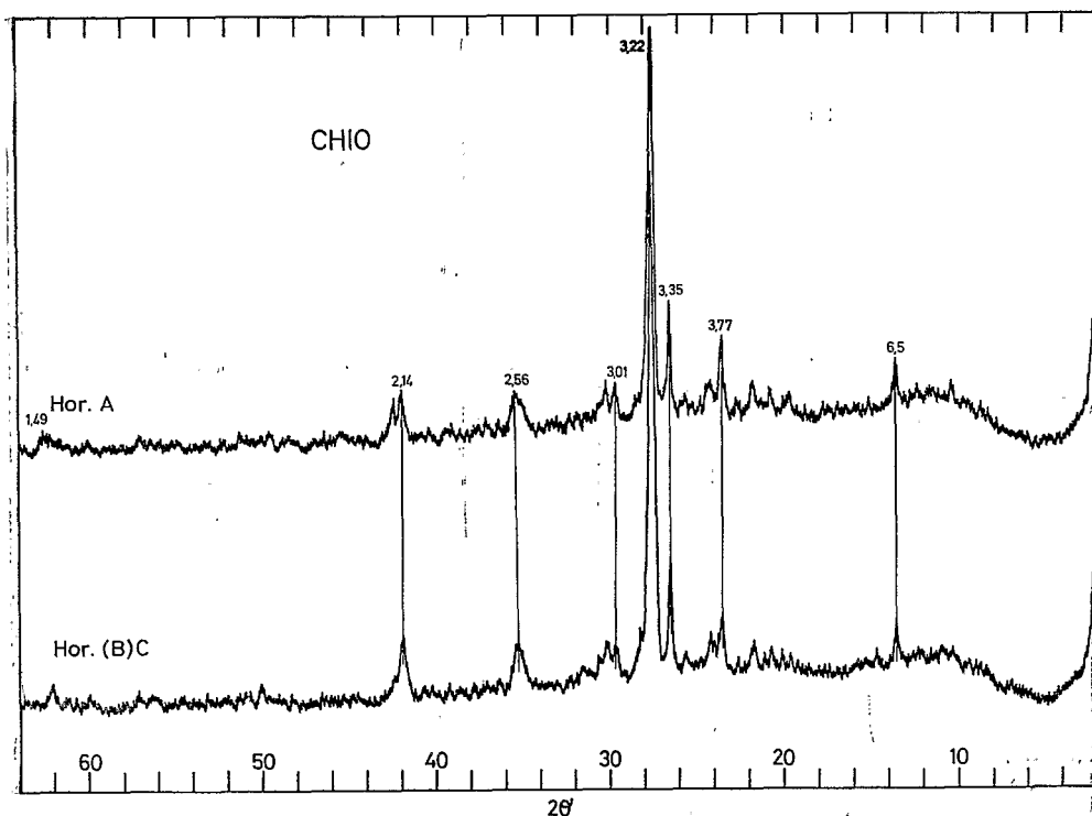
Gráfica 2.—Diagramas de difracción de rayos X, perfil «Chío» (método de Debye-Sherrer).
