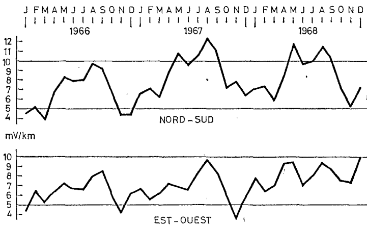
Fig. 1. Évolution annuelle de l'amplitude diurne des composantes telluriques NS et EW
