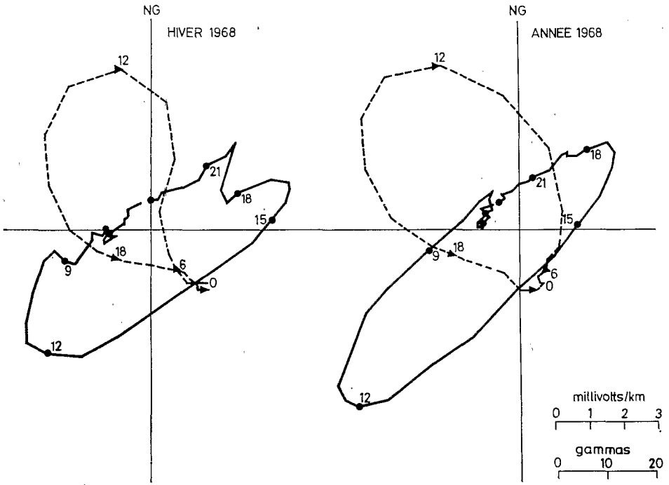
Fig. 5. Exemples de diagrammes polaires telluriques et magnétiques (moyennes saisonnière
