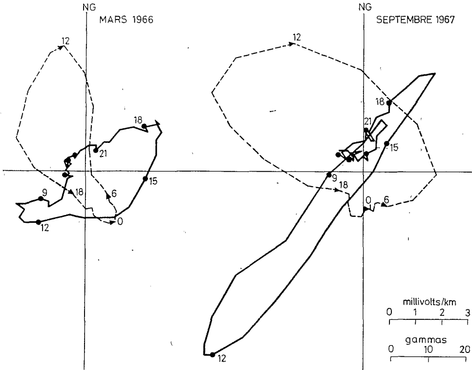
Fig. 4. Exemples de diagrammes polaires telluriques et magnétiques (moyennes mensuelles)
