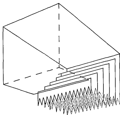
DETAIL DU SIMULATEUR DE PLUIE
