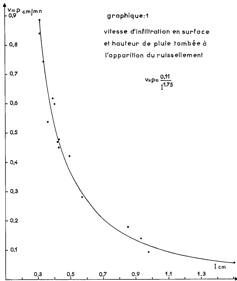
Graphique 1 — Vitesse d'infiltration en surface et hauteur de pluie tombée à l'apparition du ruissellement.
